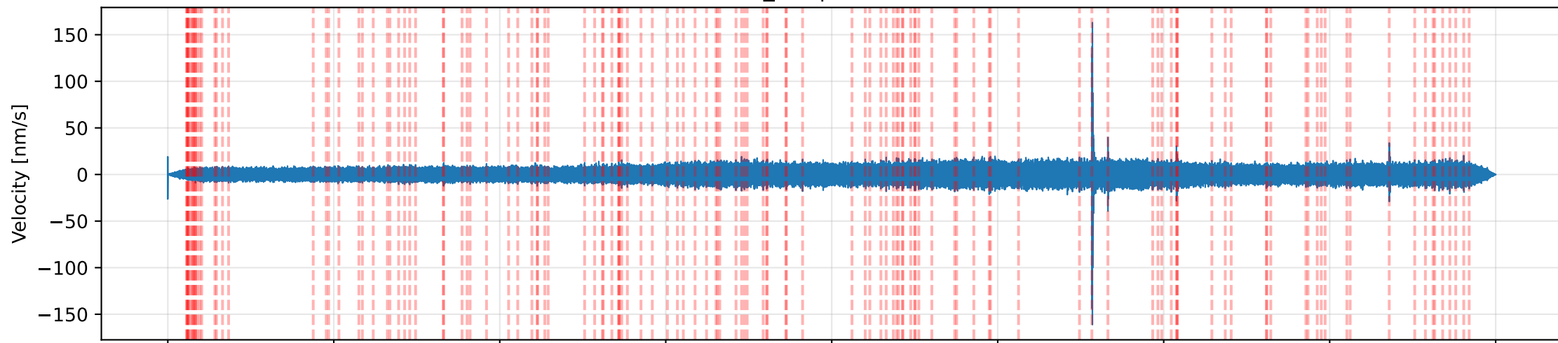
STA_LTA | 1.0-3.0Hz
