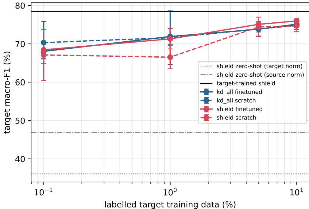
xciciot \rightarrow xciciomt, shared5
