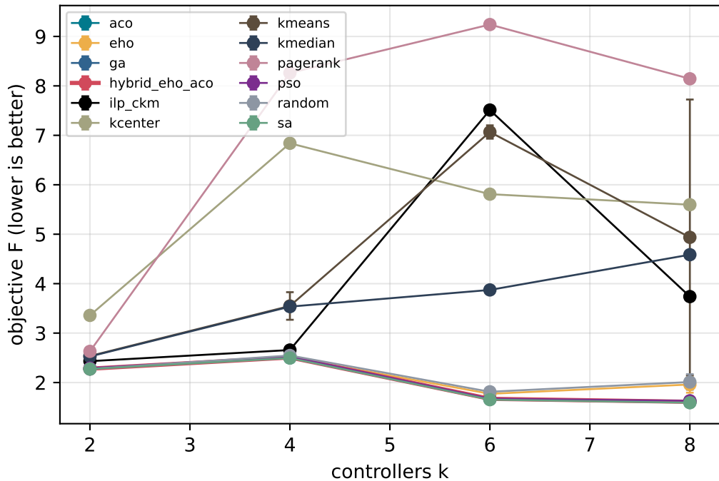
syn100, rho=0.5
