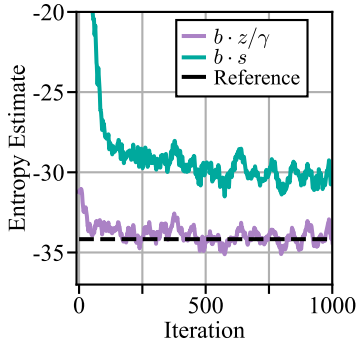
LJ Cluster
