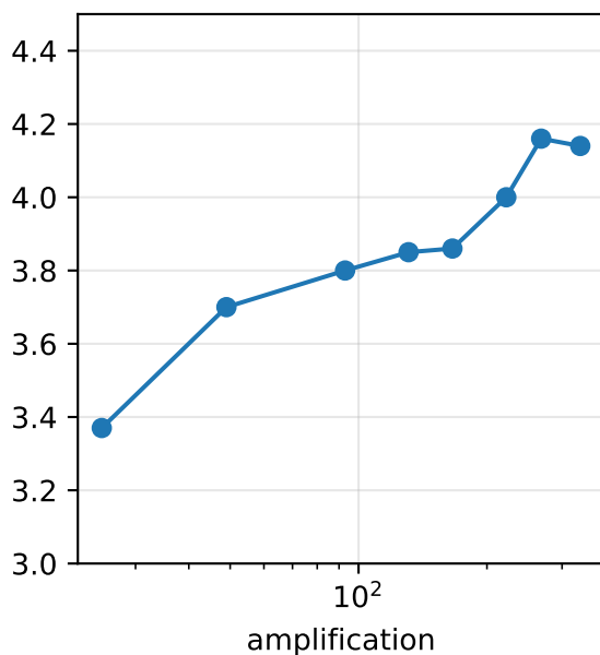
A(T-t) , T = 0.0022865
