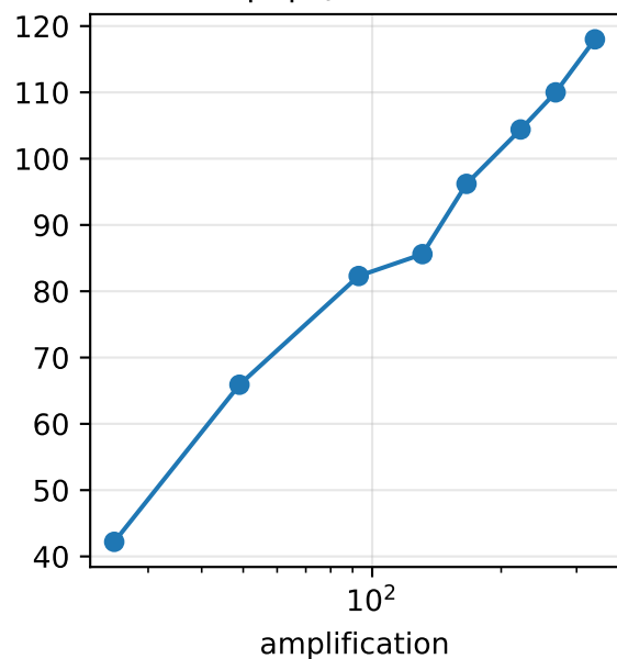
|\omega|_{\max}(T-t)
