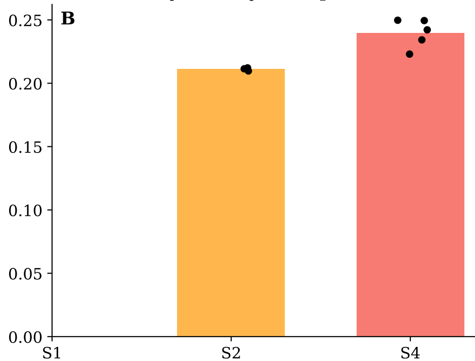
Decode Error
