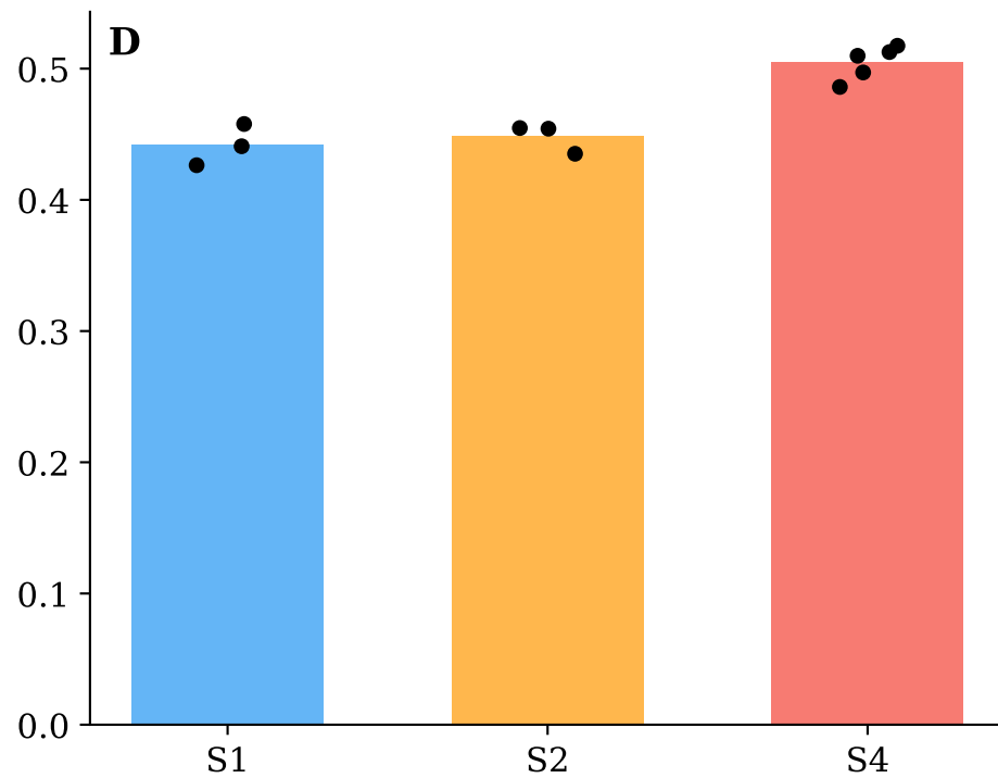
Decode Error
