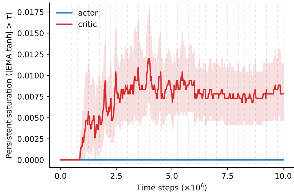
Pre-tanh 1
