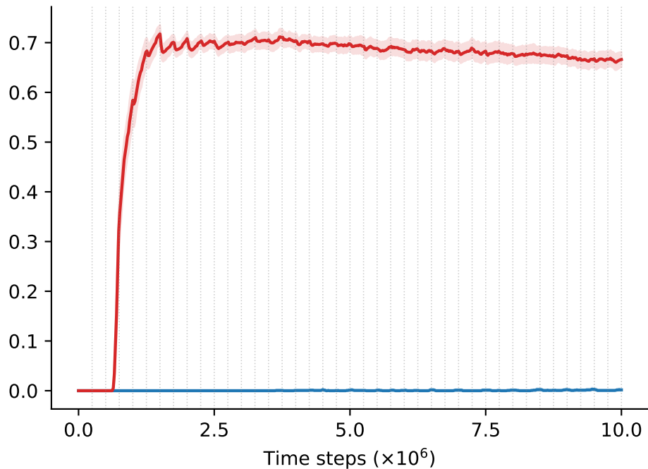
Pre-tanh 2
