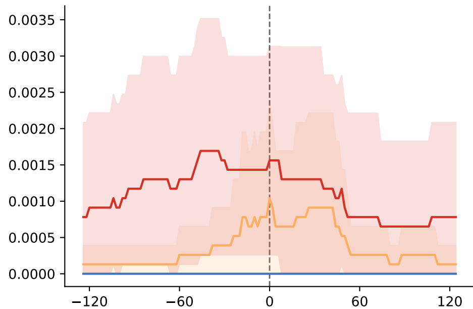
Pre-tanh 2
