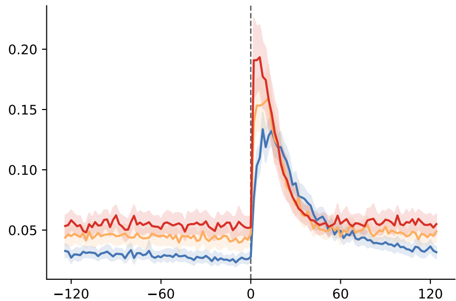
Pre-tanh 2
