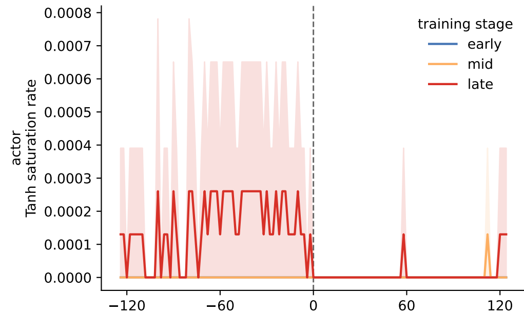
Pre-tanh 1
