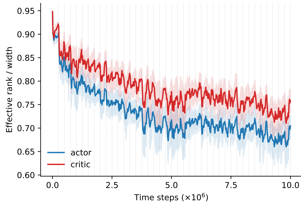
Pre-tanh 1
