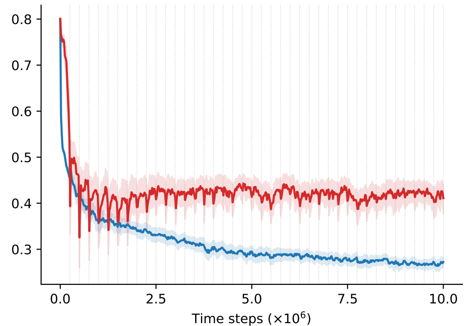
Pre-tanh 2
