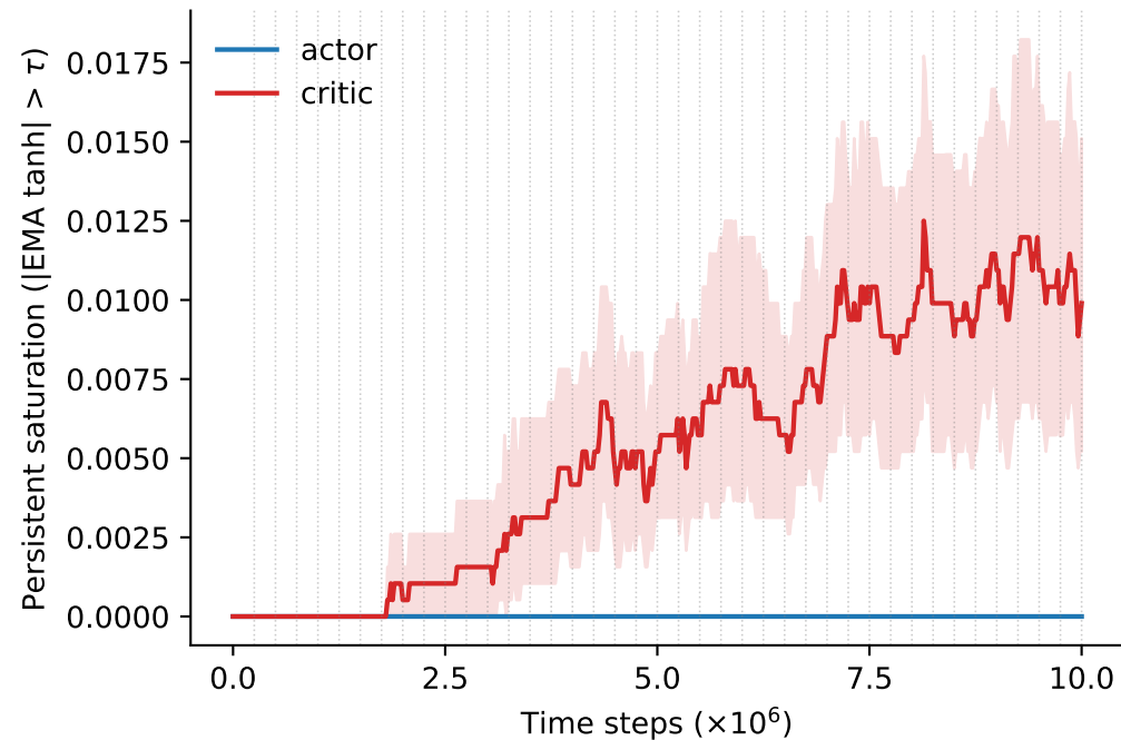
Pre-tanh 1
