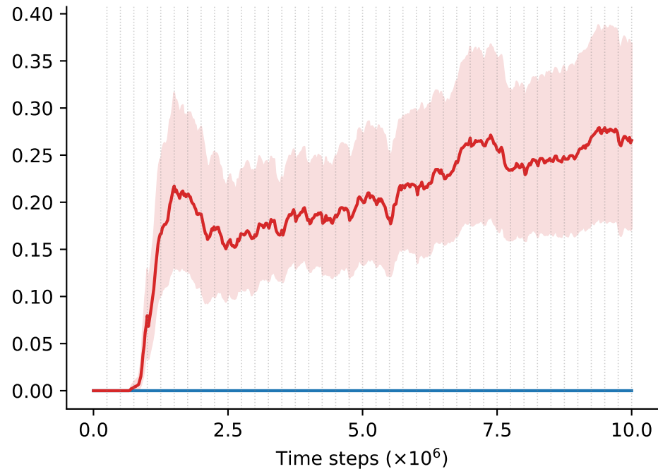
Pre-tanh 2
