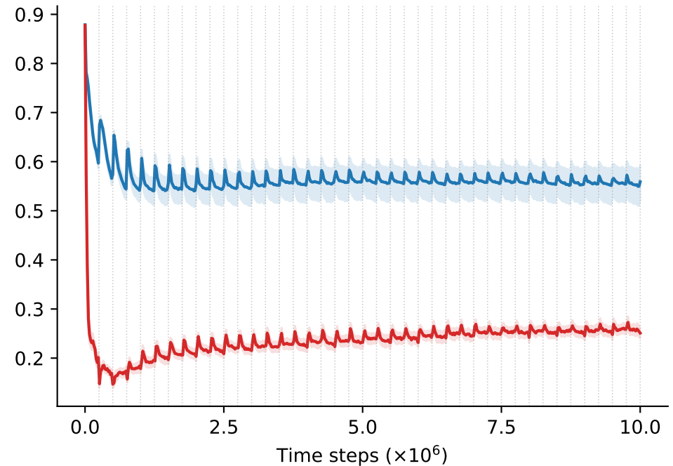
Pre-tanh 2
