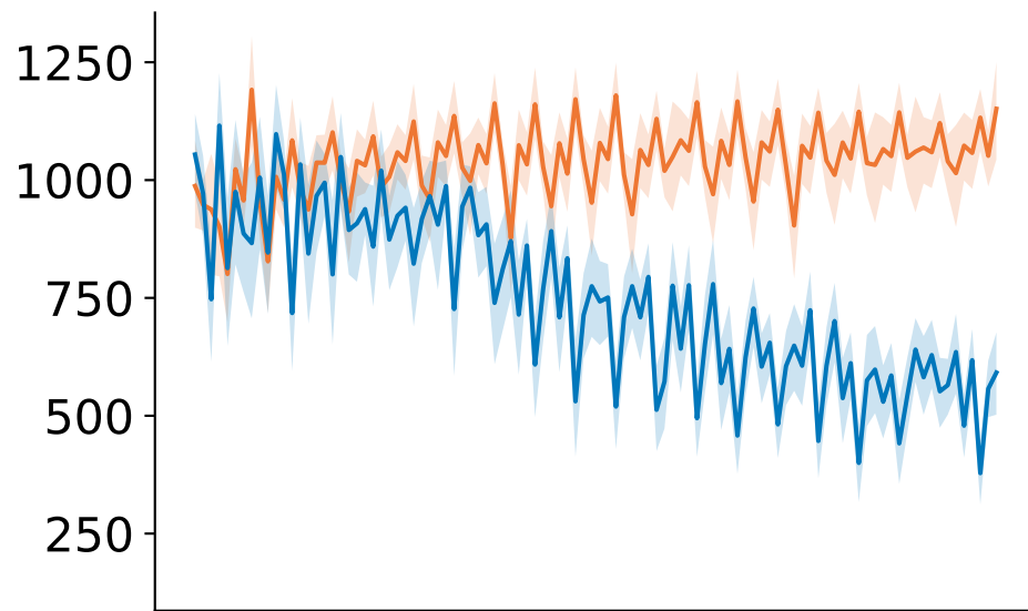
NTK Rank
