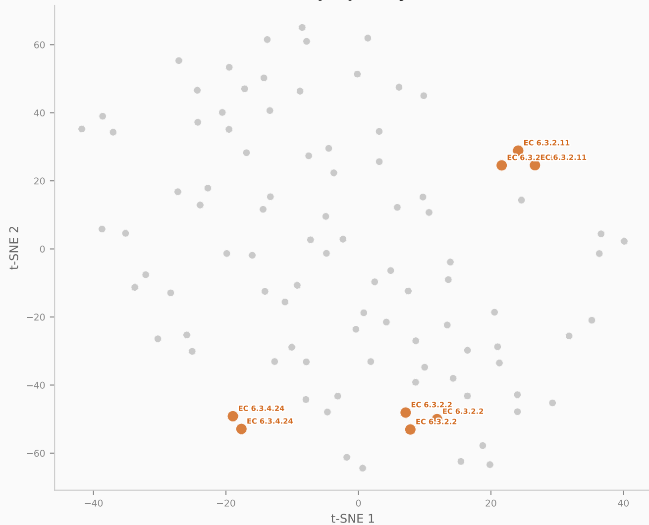
t-SNE (perplexity=24)
