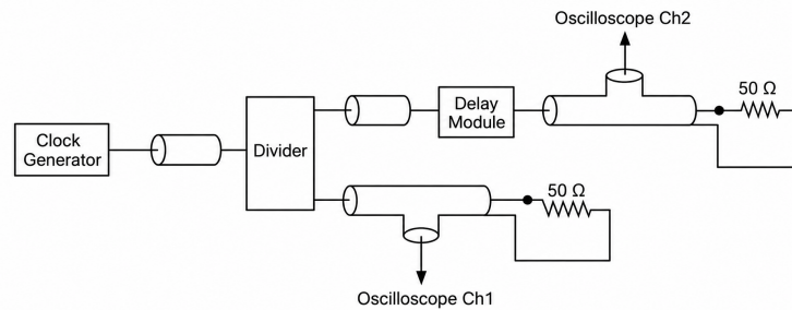
図 A.4: 遅延回路の出力の確認
