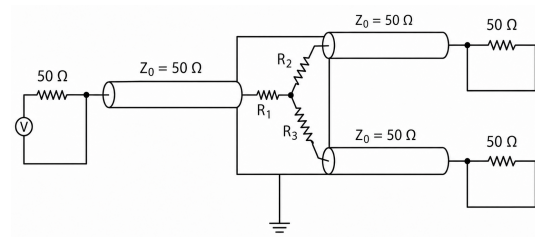
図 A.2: 電圧分割器の内部構成
