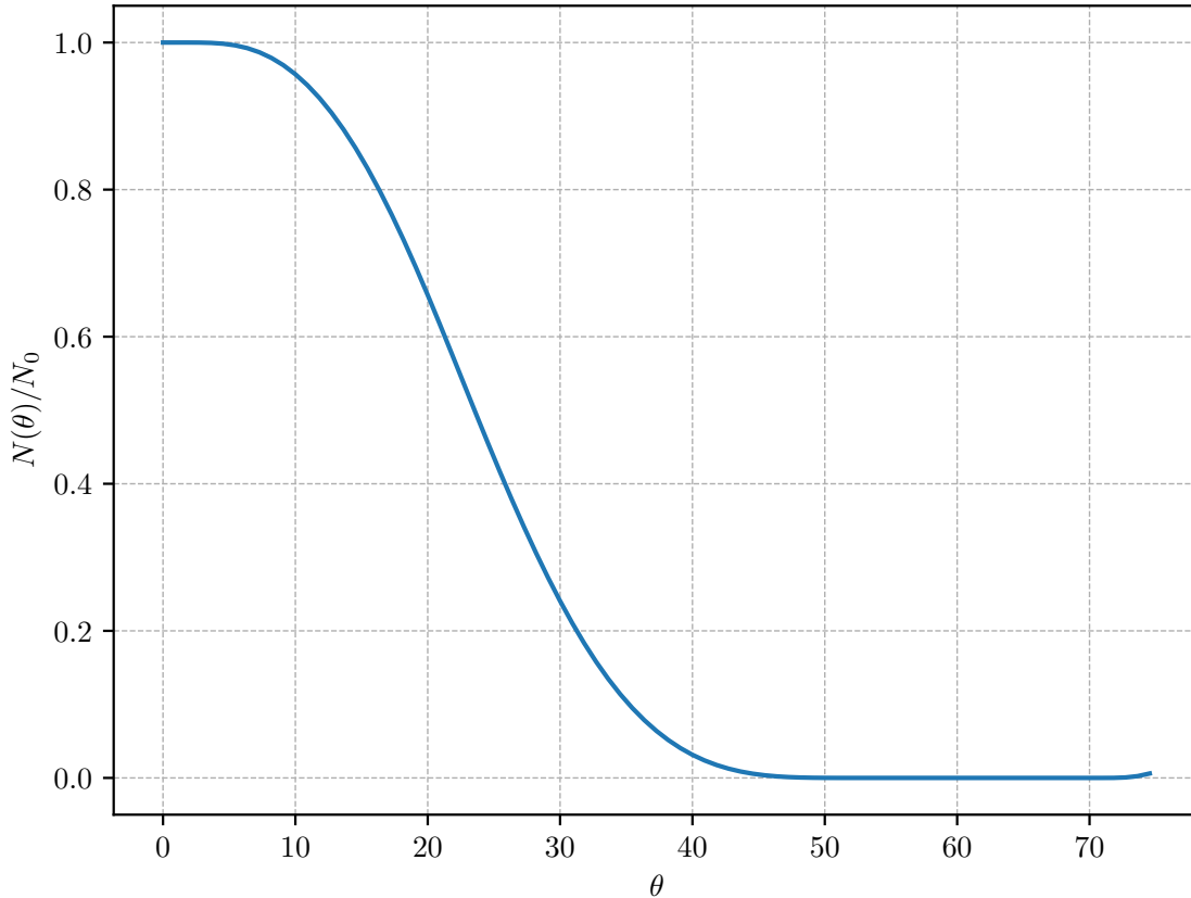
図 A.8: 数値積分から得た同時測定 of 角度分布
