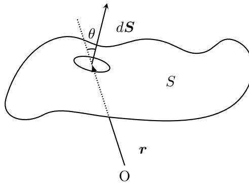
図 A.2: 曲面 S と微小面素ベクトル dS
