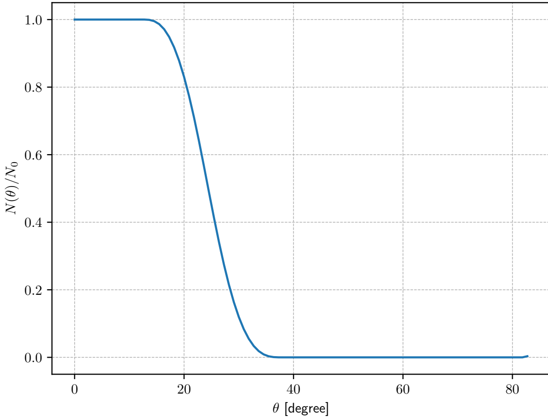
図 B.8: 数値積分から得た同時測定 of 角度分布
