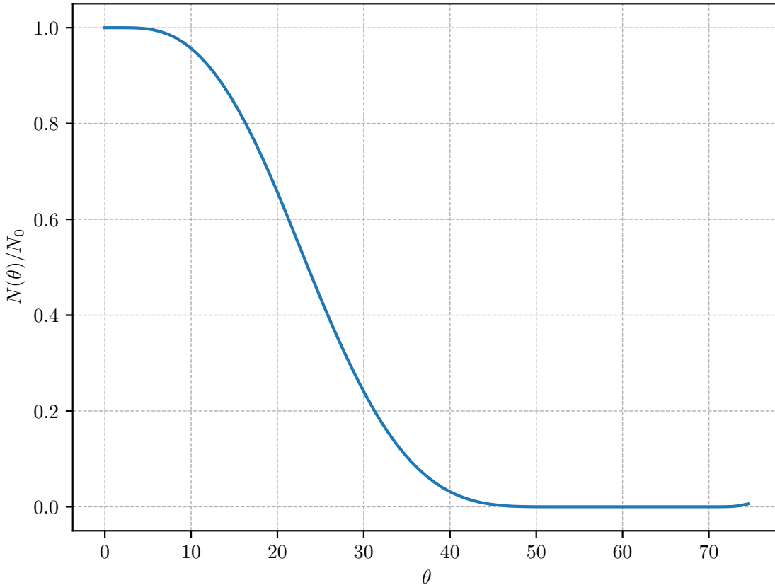
図 A.8: 数値積分から得た同時測定の角度分布
