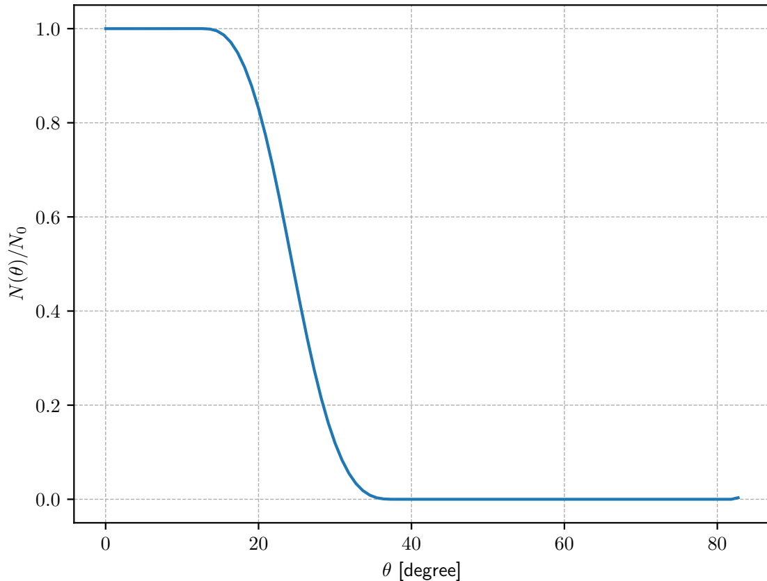
図 B.8: 数値積分から得た同時測定の角度分布
