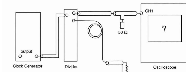
図 A.3: パルスのケーブル終端での反射の確認
