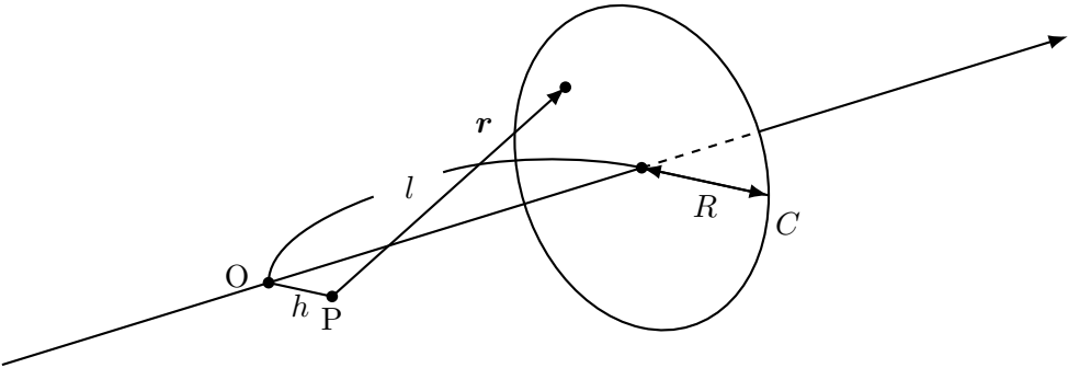
図 A.3: 斜円錐
