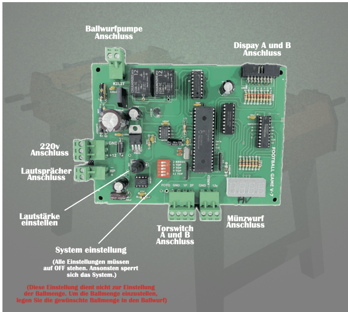
Steuerplatine des Tischkicker Pro CL – Übersicht aller Anschlüsse.
