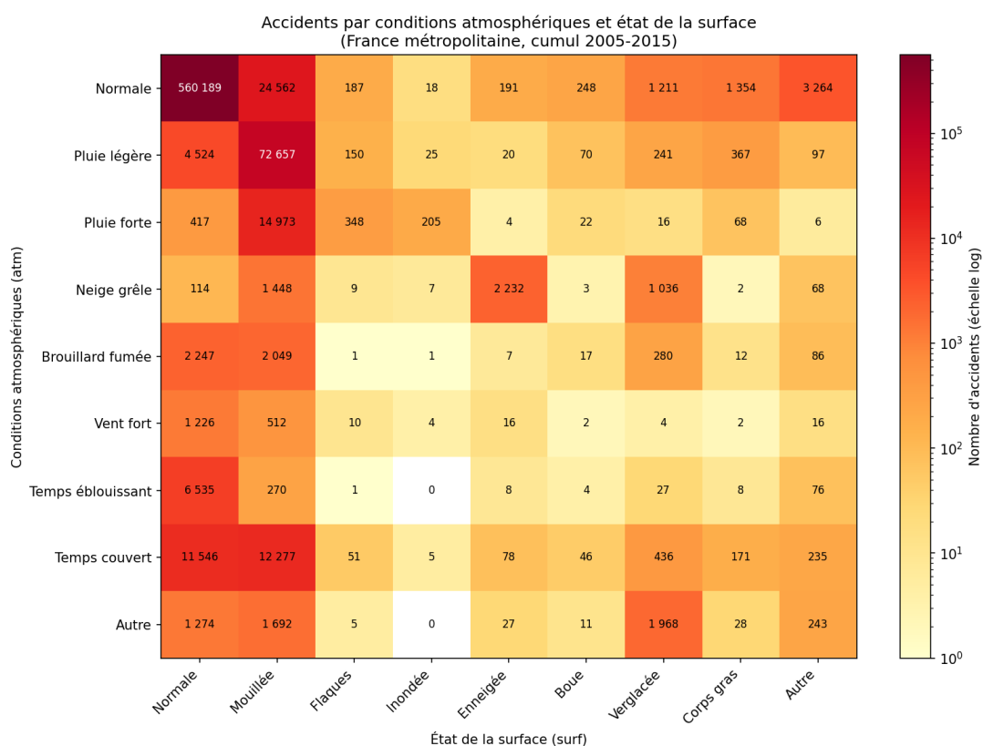
Figure 4: Q6.4 — Heatmap des accidents selon les conditions atmosphériques (atm) × état de la surface (surf), échelle logarithmique (métropole, 2005-2015).
