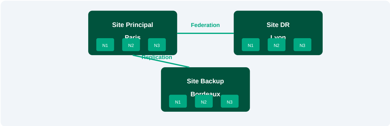
Figure 3 — Federation SimpliVity multi-sites avec replication inter-clusters
