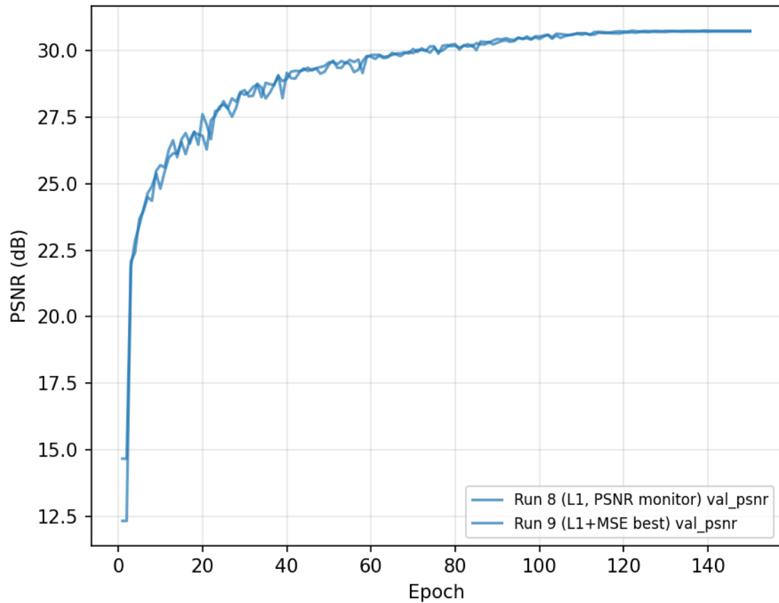
Validation PSNR
