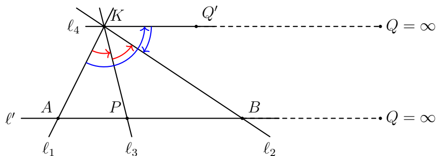
圖 5-4 線交比定理（含無窮遠點）
