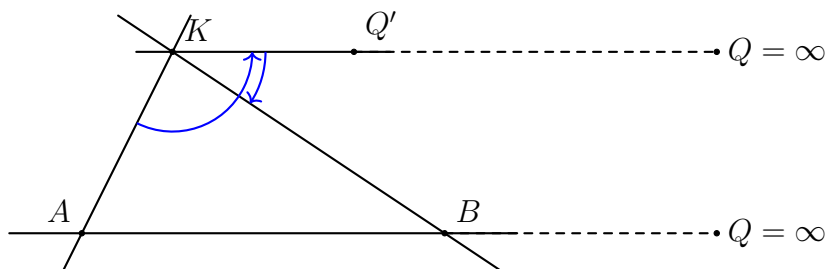
圖 5-3 有向分比定理（含無窮遠點）
