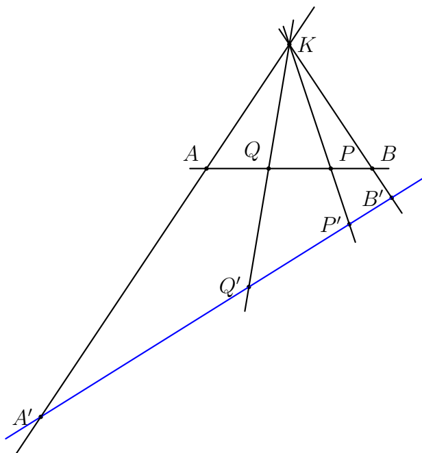
圖 4-2 線-線射影交比不變性
