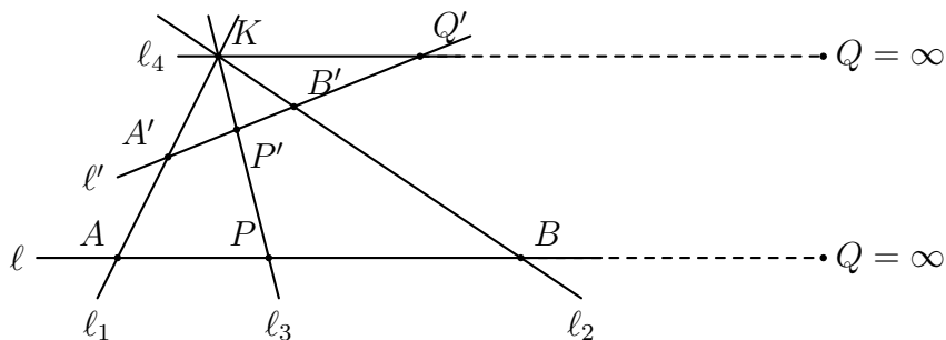
圖 5-5 性質 4 的延伸（含無窮遠點）
