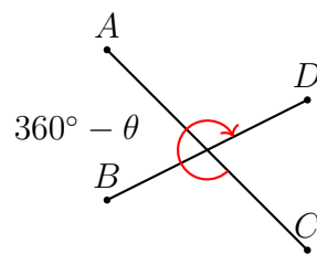
圖 2-2 \overrightarrow{OA} 順時針旋轉 360^\circ - \theta 後，與 \overrightarrow{OB} 重合（或平行）
