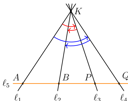
圖 4-1 交比定理
