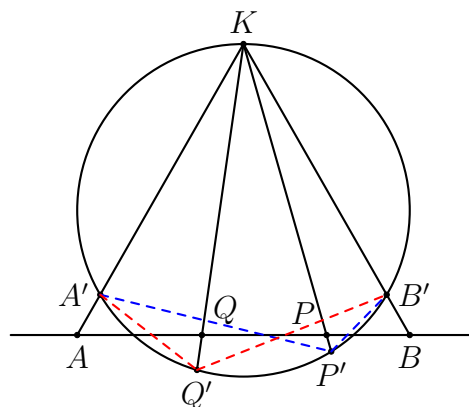
圖 4-7 線-圓射影交比不變性
