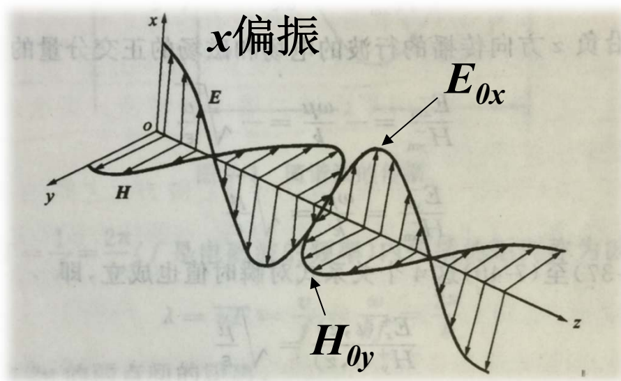
图中 z=0 处 E 和 H 相位刚好为0
