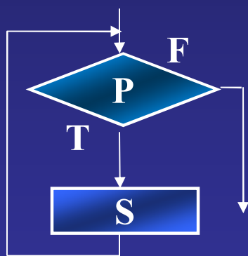
当型循环
