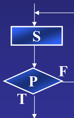
直到型循环
