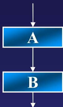
顺序结构
