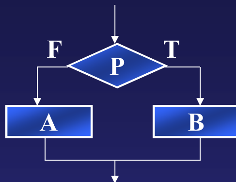
选择结构
