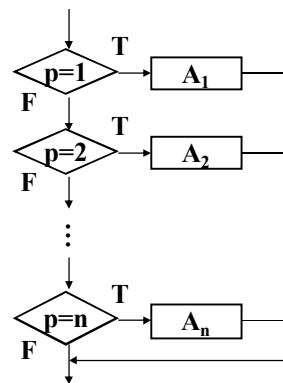
多情况选择结构 (多路选择结构)
