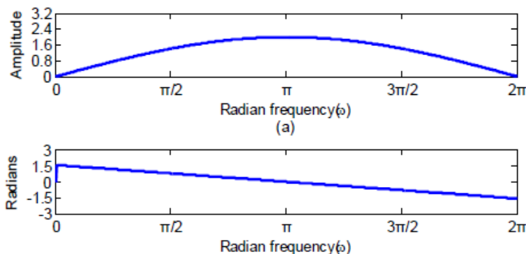
频率响应
