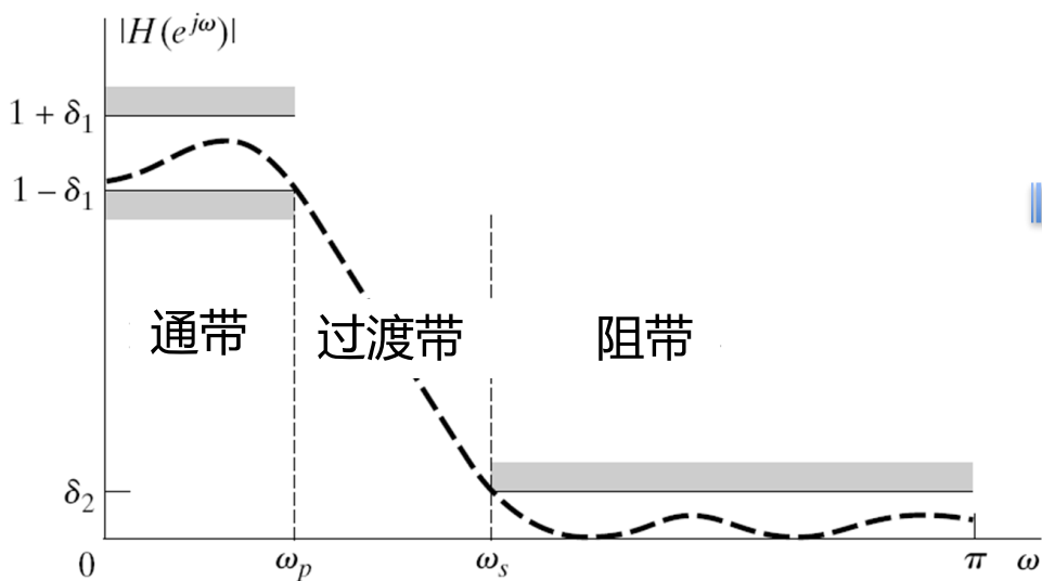
典型低通滤波器
