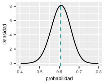
Distribución de fallecidos ( \alpha = 60.687 , \beta = 39.303 )
