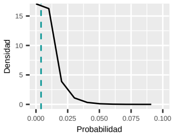
Distribución de Ind. con flores ( \alpha = 10.197 , \beta = 89.793 )
