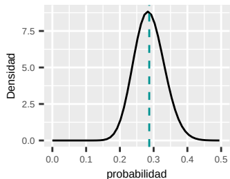
Distribución de rosetas ( \alpha = 28.71 , \beta = 71.28 )
