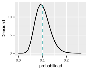
Distribución de Ind. con flores ( \alpha = 10.197 , \beta = 89.793 )
