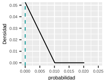
Distribución de fallecidos ( \alpha = 60.687 , \beta = 39.303 )
