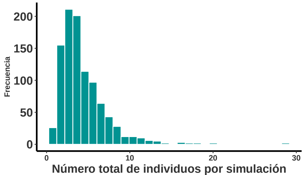
Distribución de total de individuos esperado de *Serapias con
