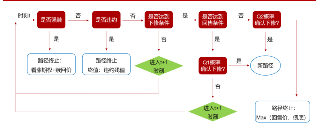
图3：LSM 转债定价模型中单条路径处理流程
