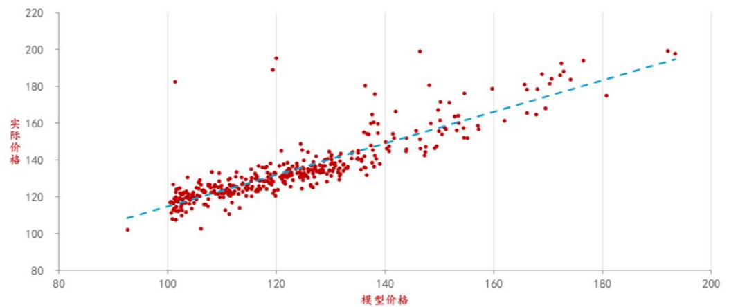
图5：LSM 转债定价模型结果与实际价格高度相关
