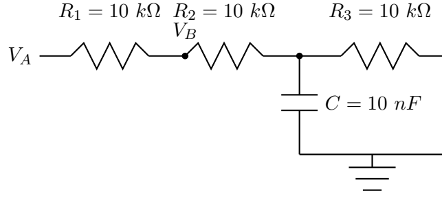
Figura 12: Circuito de prueba utilizado para las medidas de impedancia.
