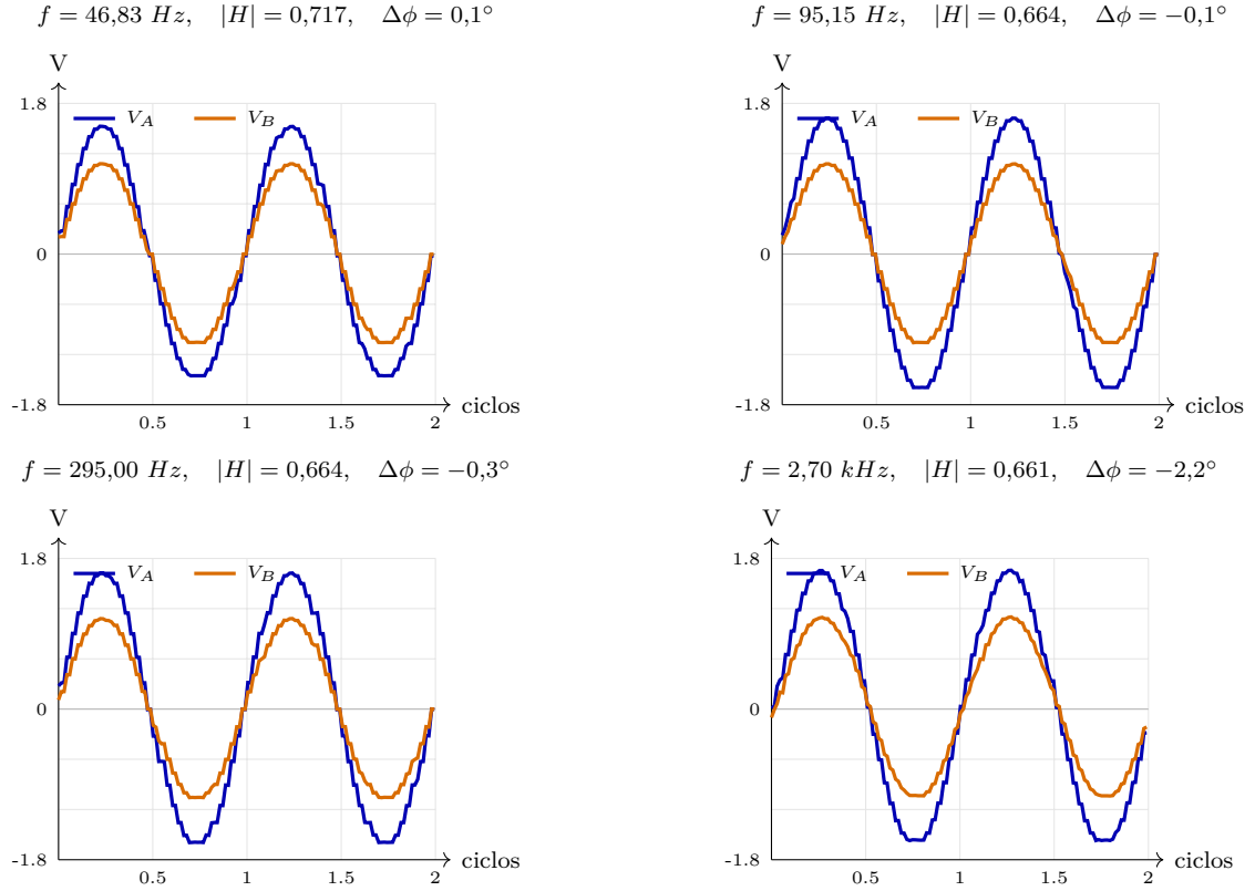
Figura 14: Formas de onda medidas a frecuencias intermedias. La escala comãn permite comparar directamente la amplitud de entrada y salida.
