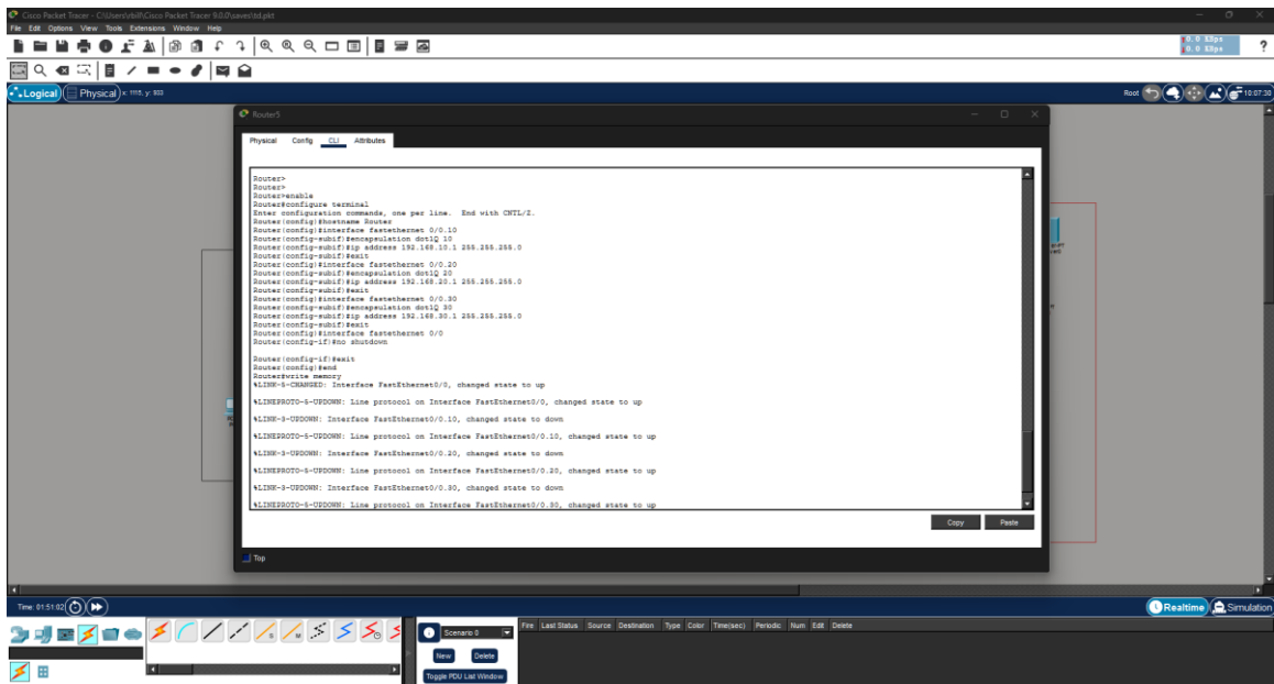
Configuration du routeur avec les sous-interfaces VLAN 10, 20 et 30.
