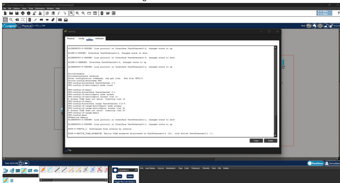
Configuration du switch SW3
