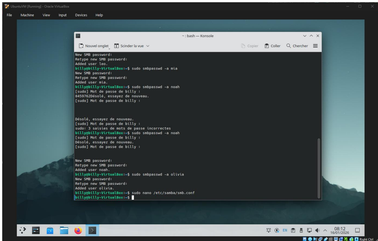
Figure 4: Creation des utilisateurs supplémentaires
