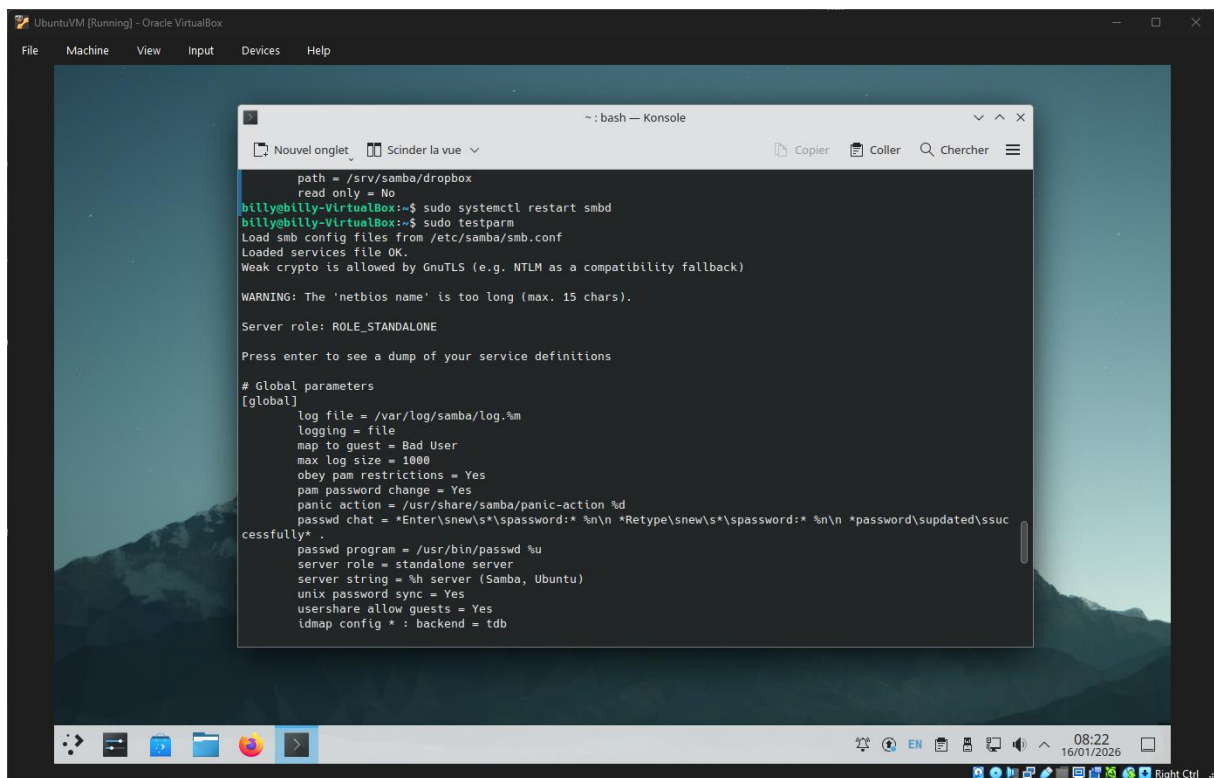
Figure 5: Verification de la configuration avec testparm
