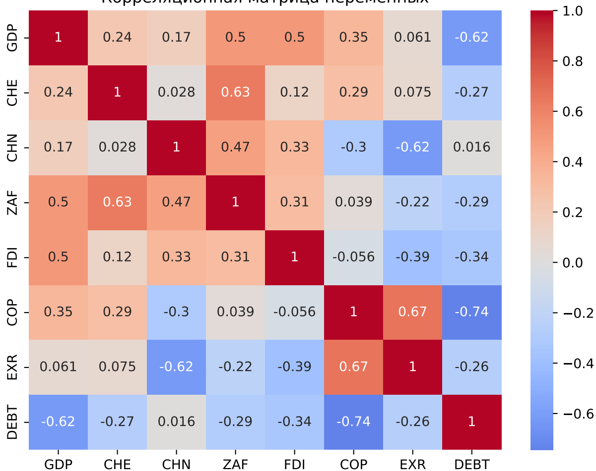
Корреляционная матрица переменных
