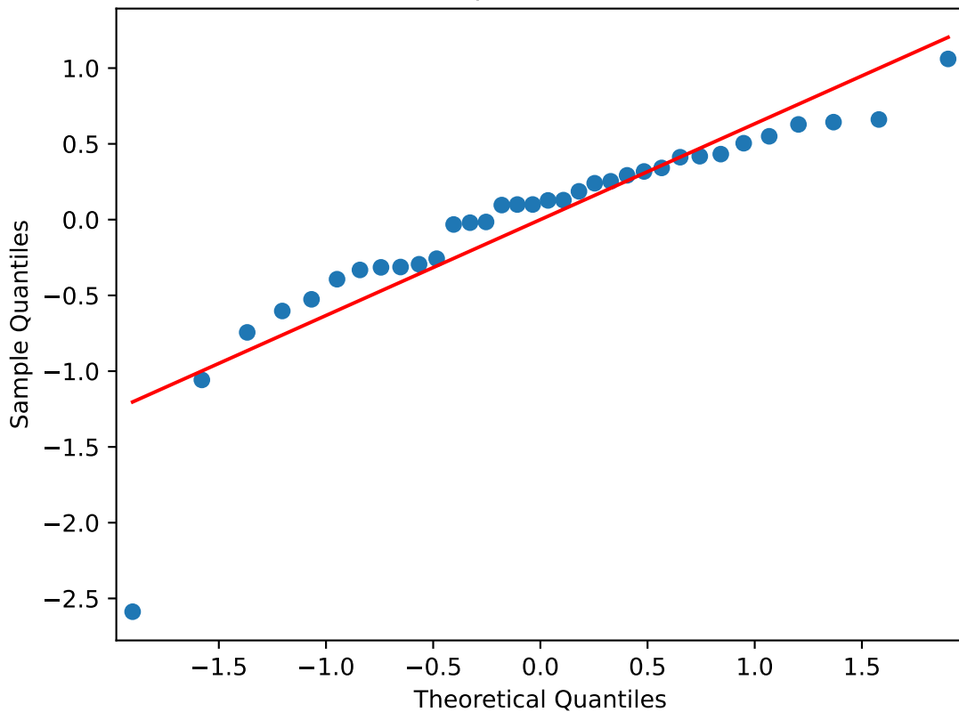
Q-Q plot остатков
