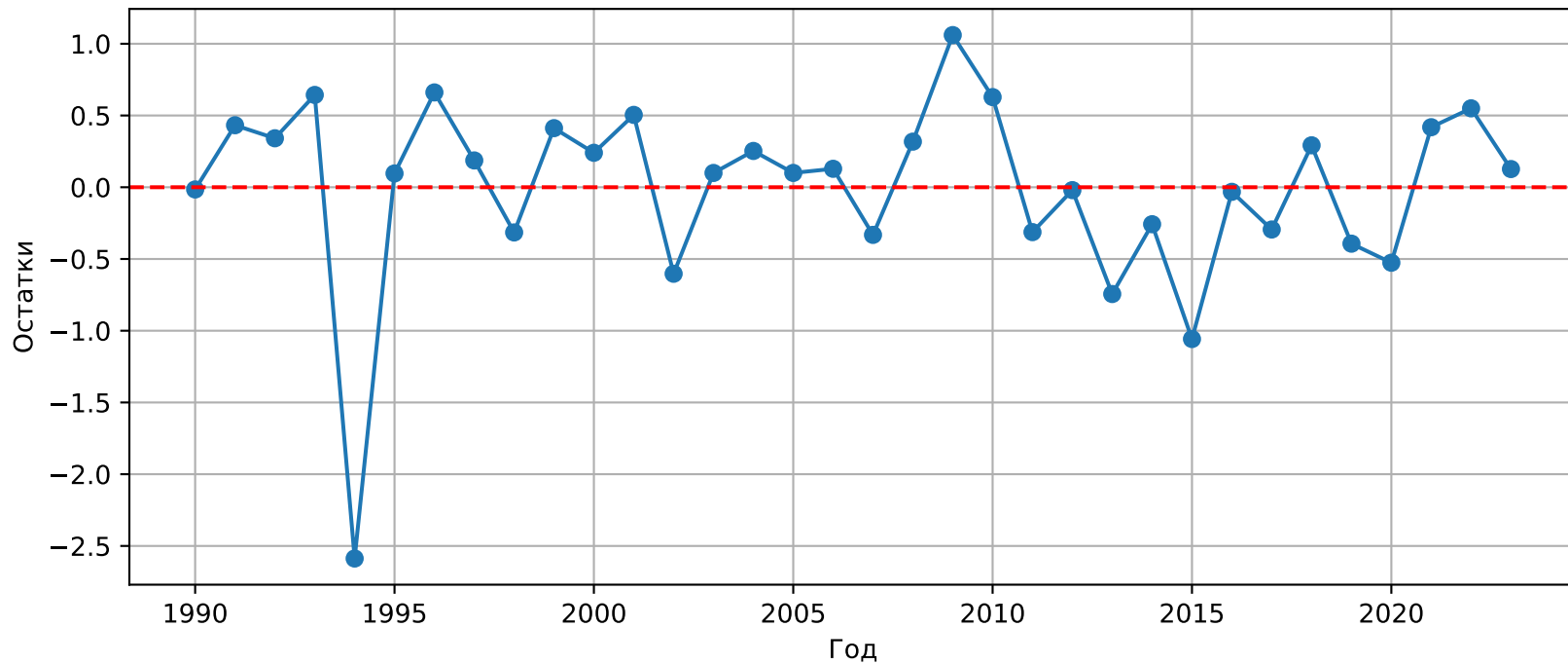
Остатки модели по годам
