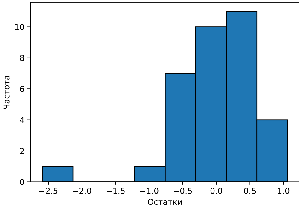
Гистограмма остатков
