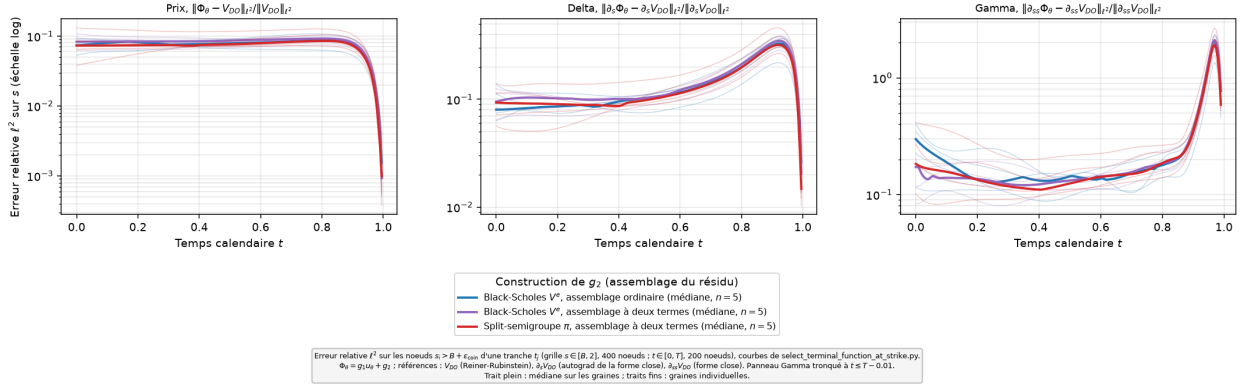
FIGURE 1 – [MESURÉ] Figure « erreur vs temps » du rapport de sélection, répliquée à cinq graines par le même script ( select_terminal_function_at_strike.py ). Erreur relative \ell^2 sur les noeuds s_i > B + \varepsilon_{\text{coin}} = 0.7 d'une tranche t_j (grille s \in [B, 2] , 400 noeuds; t \in [0, T] , 200 noeuds), courbes de select_terminal_function_at_strike.py . \Phi_\theta = g_1 u_\theta + g_2 ; références : V_{DO} (Reiner-Rubinstein), \Delta V_{DO} (intégral de la forme close), \Delta u_\theta V_{DO} (forme close), panneau Gamma tronqué à t \leq T - 0.01 . Trait plein : médiane sur les graines ; traits fins : graines individuelles.
