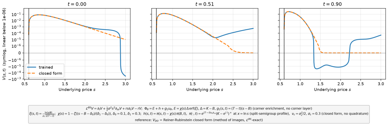
FIGURE 50 – Coupes V(s, t) à t \in \{0, 0.5, 0.9\} , échelle symlog (solution entraînée en trait plein, forme fermée en tirets; trait vertical : s = B ). enrichissement du coin ( \chi \Delta \operatorname{erf}(\xi) ), profil split-semigroupe.
