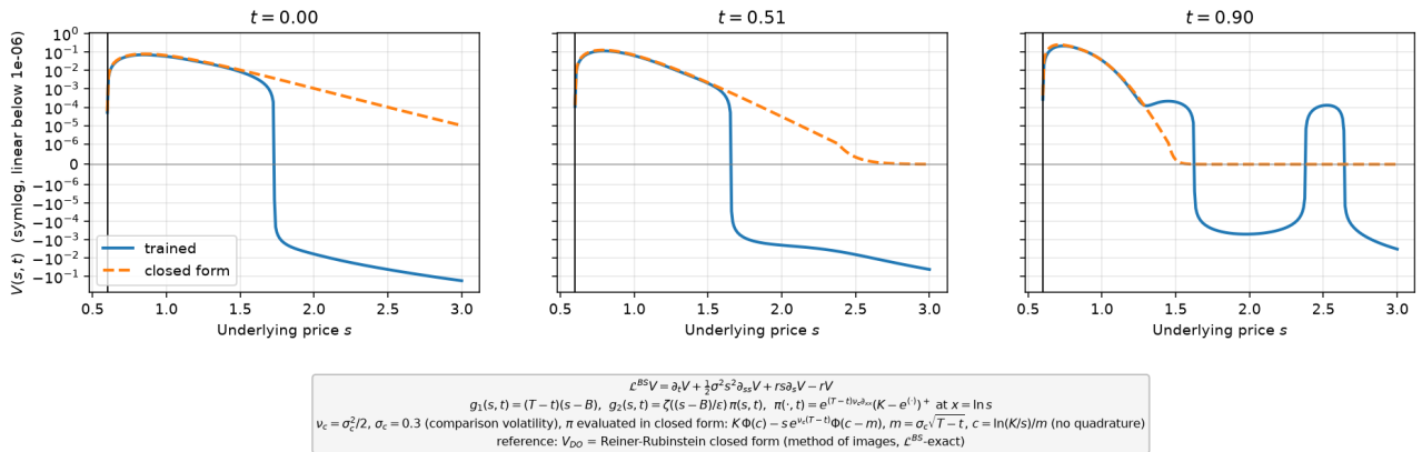
FIGURE 33 – Coupes V(s, t) à t \in \{0, 0.5, 0.9\} , échelle symlog (solution entraînée en trait plein, forme fermée en tirets; trait vertical : s = B ). .
