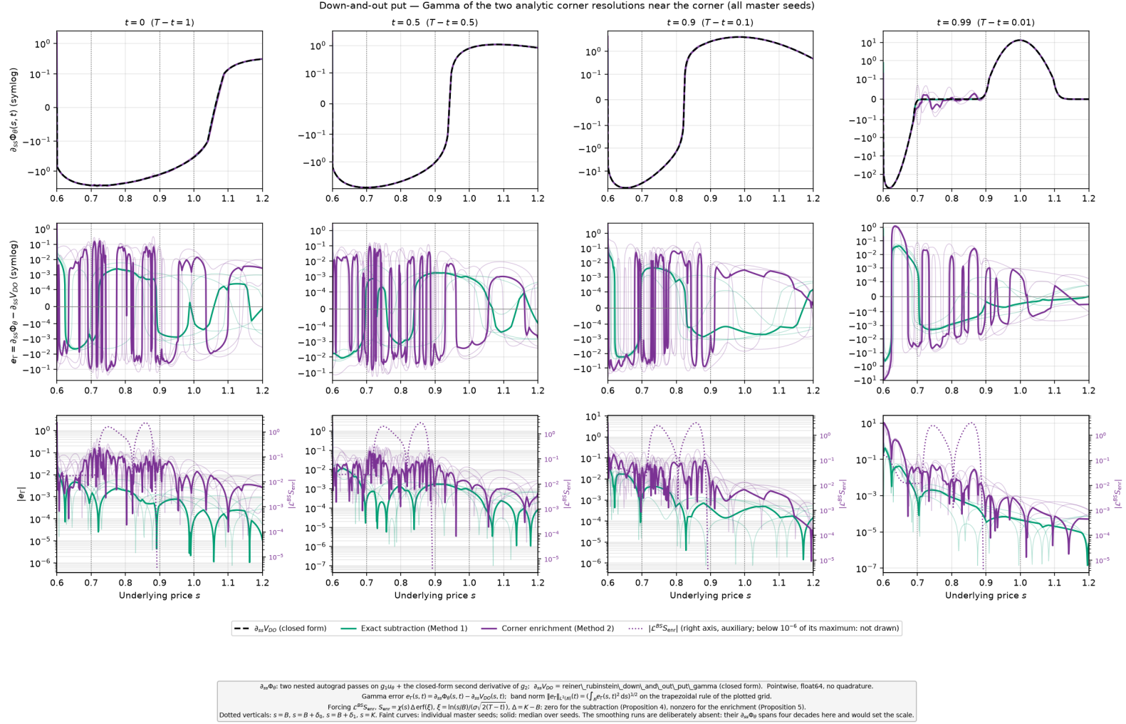
FIGURE 23 – Ligne du haut : \partial_{ss}\Phi_\theta(s, t) des deux traitements (médiane sur les graines en trait épais, graines individuelles en trait fin) et \partial_{ss}V_{DO} en tirets noirs. Ligne du milieu : l'erreur signée e_T , en échelle symlog. Ligne du bas : |e_T| en échelle logarithmique, avec |L^{BS}S_{enr}| superposé en pointillé sur l'axe de droite. La lecture : l'erreur de Gamma de l'enrichissement oscille entre la barrière et s = B + \delta_1 = 0.9 , exactement le support du forçage, et rejoint celle de la soustraction au-delà.
