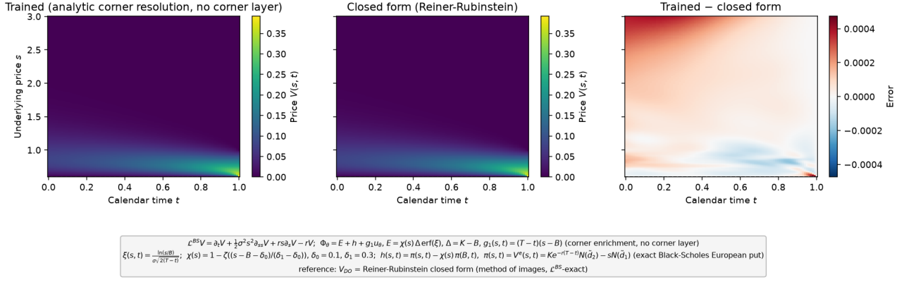
FIGURE 46 – Surface de prix : solution entraînée, forme fermée, différence. enrichissement du coin ( \chi\Delta \text{erf}(\xi) ), profil Black-Scholes V^e .
