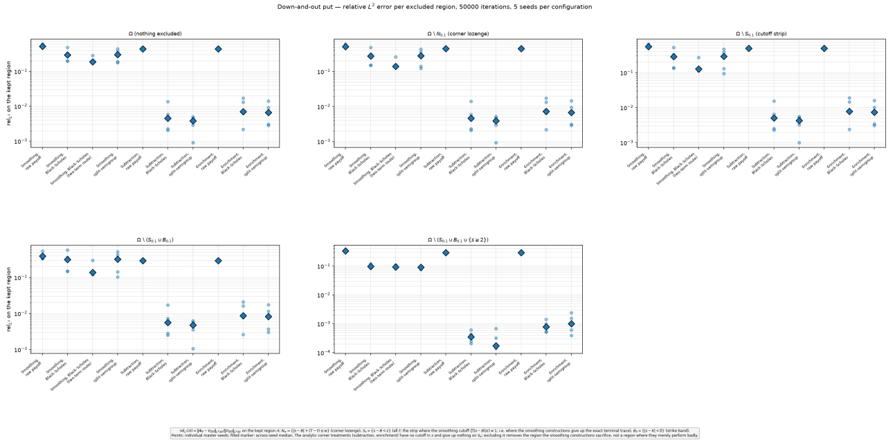
FIGURE 17 – rel_{L^2}(A) = \|\Phi_\theta - V_{DO}\|_{L^2(A)} / \|V_{DO}\|_{L^2(A)} sur la région conservée A , un panneau par région exclue ; points : graines individuelles, losange plein : médiane sur les graines.
