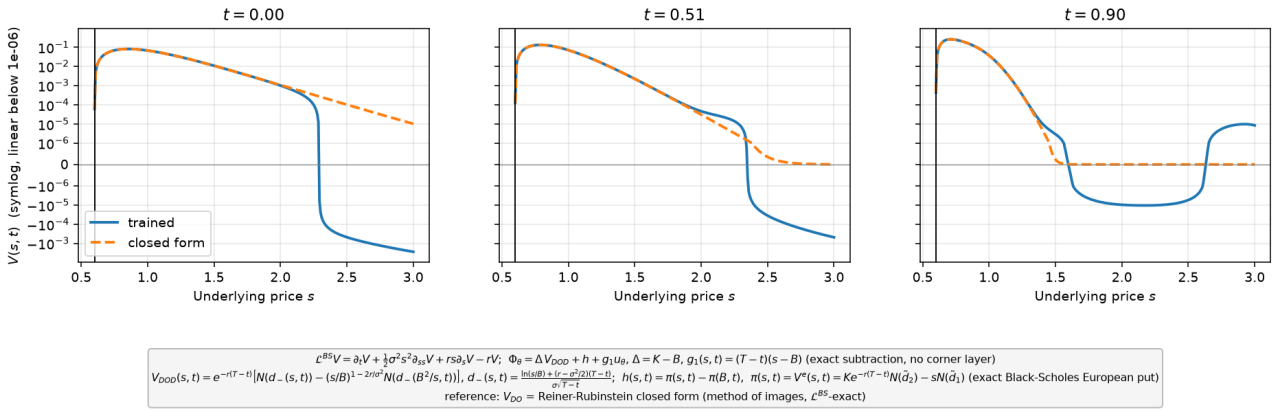
FIGURE 38 – Coupes V(s, t) à t \in \{0, 0.5, 0.9\} , échelle symlog (solution entraînée en trait plein, forme fermée en tirets ; trait vertical : s = B ). soustraction exacte ( \Delta V_{DOD} ), profil Black-Scholes V^e .
