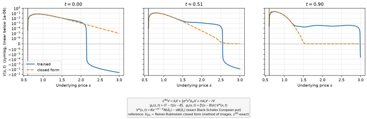
FIGURE 31 – Coupes V(s, t) à t \in \{0, 0.5, 0.9\} , échelle symlog (solution entraînée en trait plein, forme fermée en tirets; trait vertical : s = B ). .
