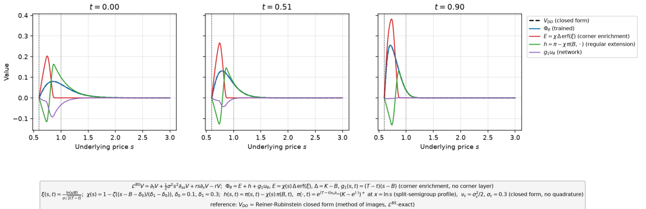
FIGURE 51 – Décomposition de l'estimateur : partie singulière en forme fermée, extension régulière h , réseau g_1 u_\theta , total, contre V_{DO} . enrichissement du coin ( \chi \Delta \operatorname{erf}(\xi) ), profil split-semigroupe.
