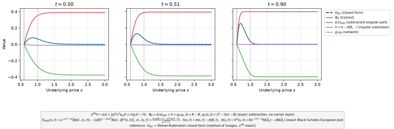
FIGURE 39 – Décomposition de l'estimateur : partie singulière en forme fermée, extension régulière h , réseau g_1 u_\theta , total, contre V_{DO} . soustraction exacte ( \Delta V_{DOD} ), profil Black-Scholes V^e .
