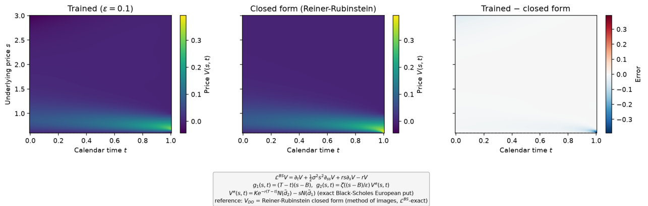
FIGURE 30 – Surface de prix : solution entraînée, forme fermée, différence. .
