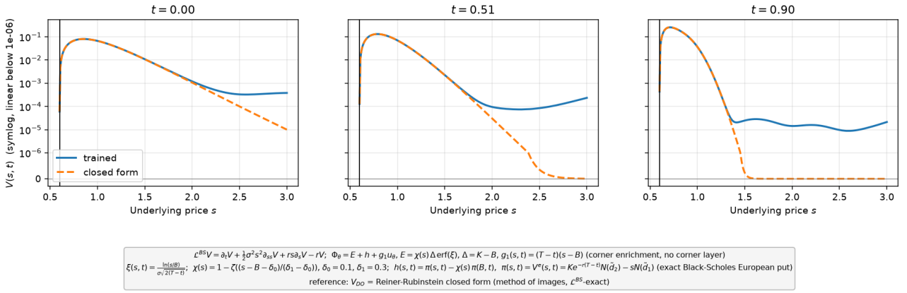
FIGURE 47 – Coupes V(s, t) à t \in \{0, 0.5, 0.9\} , échelle symlog (solution entraînée en trait plein, forme fermée en tirets ; trait vertical : s = B ). enrichissement du coin ( \chi\Delta \text{erf}(\xi) ), profil Black-Scholes V^e .
