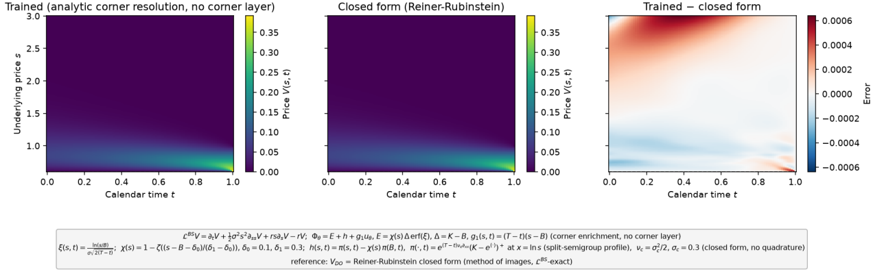
FIGURE 49 – Surface de prix : solution entraînée, forme fermée, différence. enrichissement du coin ( \chi \Delta \operatorname{erf}(\xi) ), profil split-semigroupe.
