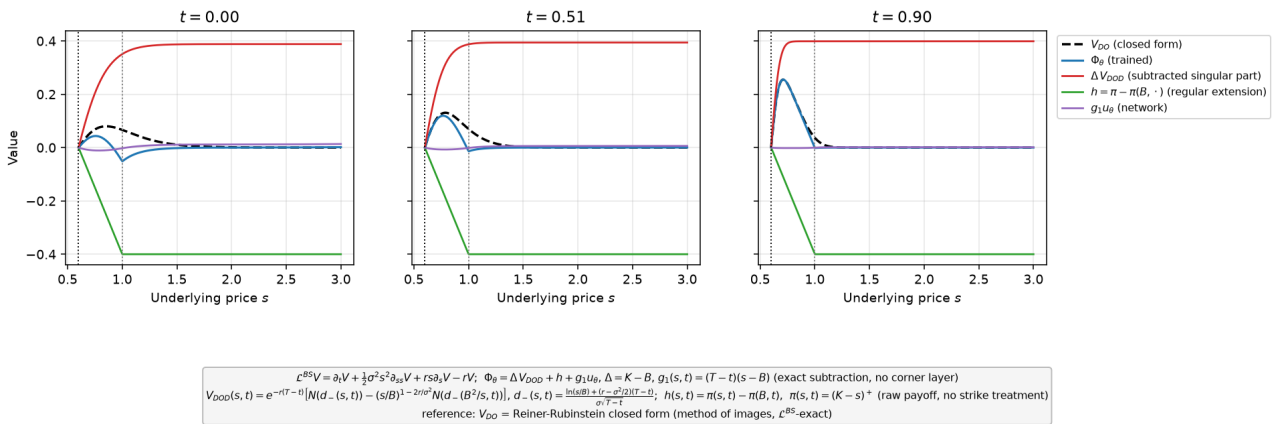
FIGURE 36 – Décomposition de l'estimateur : partie singulière en forme fermée, extension régulière h , réseau g_1 u_\theta , total, contre V_{DO} . soustraction exacte ( \Delta V_{DOD} ), profil payoff brut (contrôle négatif).
