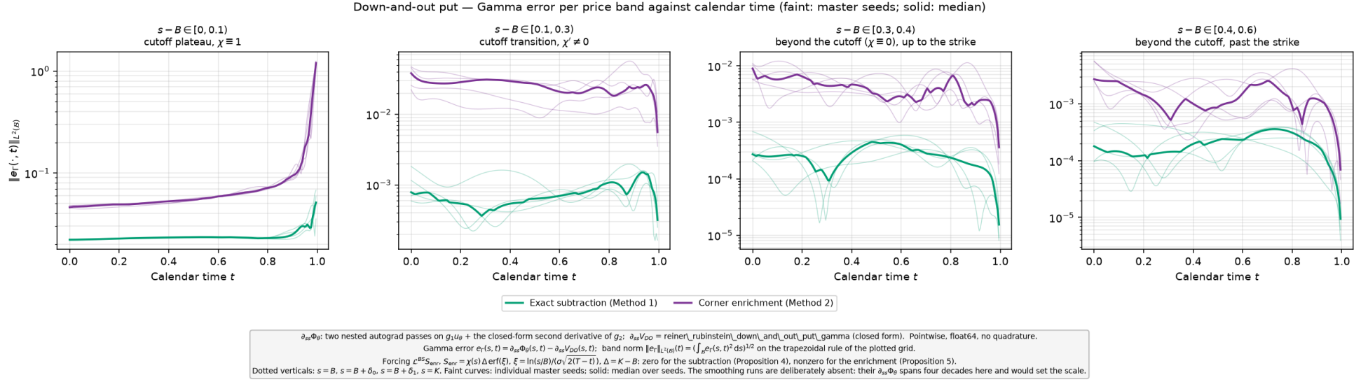
FIGURE 25 – Norme L^2 en s de l’erreur de Gamma sur chaque bande, en fonction du temps calendaire ; traits fins : graines individuelles. L’écart entre les deux traitements est reproductible sur les cinq graines (les faisceaux ne se croisent pas dans les deux premières bandes), donc il vient de la construction et non du bruit d’optimisation.
