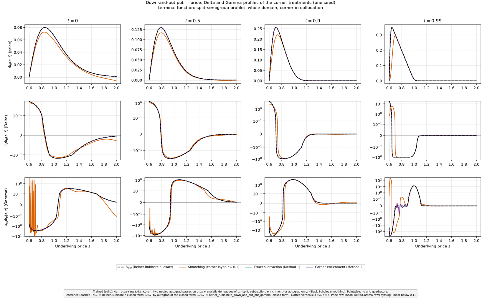
FIGURE 9 – Lignes : \Phi_\theta(s, t) , \partial_s \Phi_\theta(s, t) , \partial_{ss} \Phi_\theta(s, t) ; colonnes : t \in \{0, 0.5, 0.9, 0.99\} ; forme fermée en tirets noirs. Prix en échelle linéaire; \Delta et \Gamma en échelle symlog (linéaire sous 0.1, logarithmique au-delà, des deux côtés de zéro).
