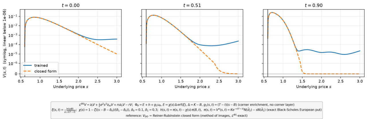
FIGURE 30 – Coupes V(s, t) à t \in \{0, 0.5, 0.9\} , échelle symlog (solution entraînée en trait plein, forme fermée en tirets; trait vertical : s = B ). enrichissement du coin ( \chi \Delta \text{erf}(\xi) ), profil Black-Scholes V^e .
