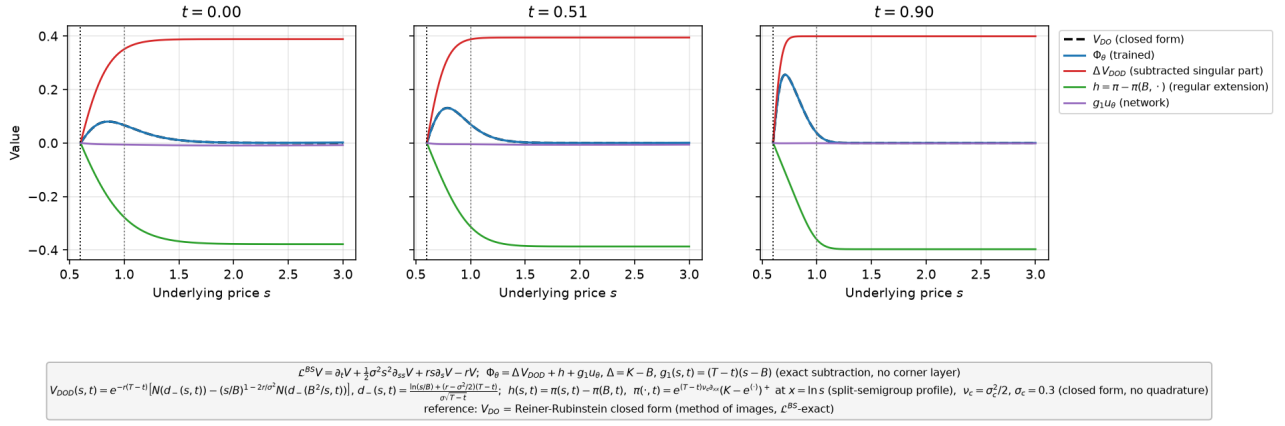
FIGURE 25 – Décomposition de l'estimateur : partie singulière en forme fermée, extension régulière h , réseau g_1 u_\theta , total, contre V_{D0} . soustraction exacte ( \Delta V_{D0D} ), profil split-semigroupe.
