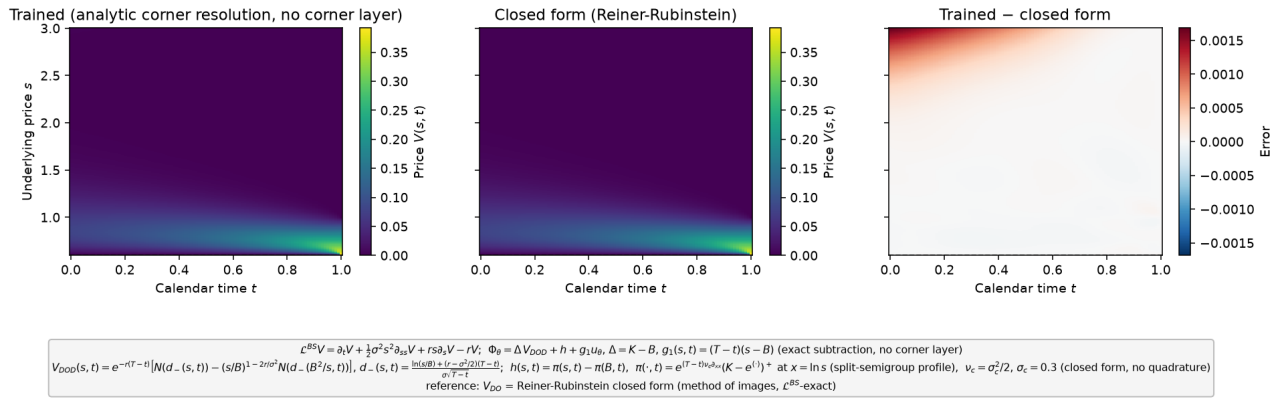
FIGURE 23 – Surface de prix : solution entraînée, forme fermée, différence. soustraction exacte ( \Delta V_{D0D} ), profil split-semigroupe.
