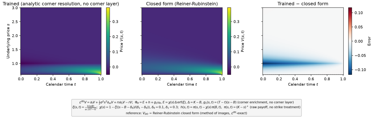
FIGURE 26 – Surface de prix : solution entraînée, forme fermée, différence. enrichissement du coin ( \chi \Delta \text{erf}(\xi) ), profil payoff brut (contrôle négatif).
