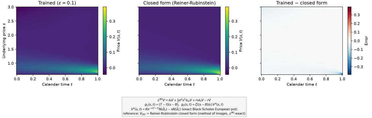
FIGURE 13 – Surface de prix : solution entraînée, forme fermée, différence. .
