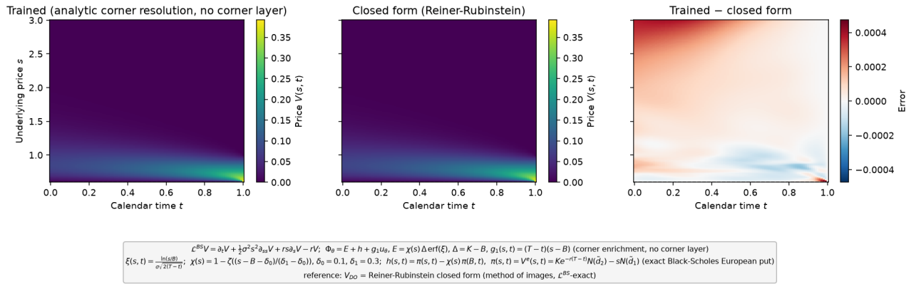
FIGURE 29 – Surface de prix : solution entraînée, forme fermée, différence. enrichissement du coin ( \chi \Delta \text{erf}(\xi) ), profil Black-Scholes V^e .
