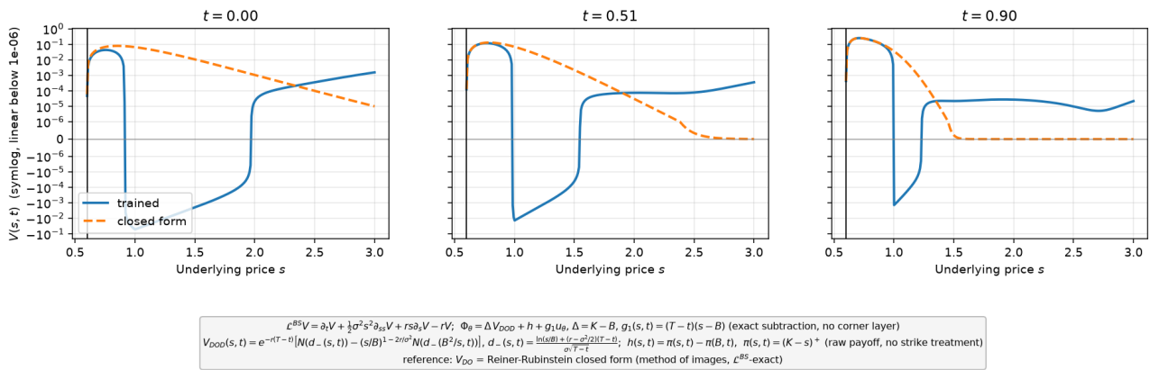
FIGURE 18 – Coupes V(s, t) à t \in \{0, 0.5, 0.9\} , échelle symlog (solution entraînée en trait plein, forme fermée en tirets; trait vertical : s = B ). soustraction exacte ( \Delta V_{DOD} ), profil payoff brut (contrôle négatif).
