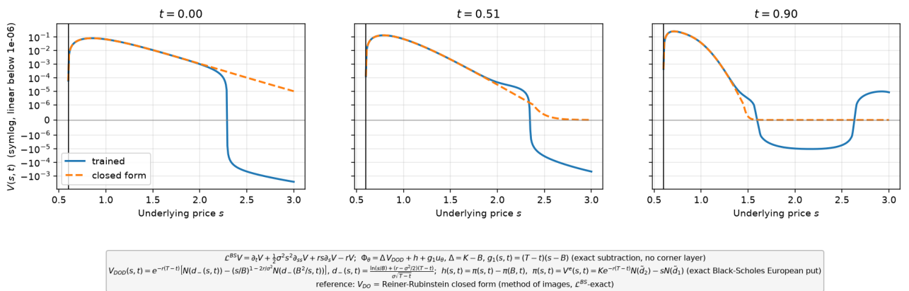
FIGURE 21 – Coupes V(s, t) à t \in \{0, 0.5, 0.9\} , échelle symlog (solution entraînée en trait plein, forme fermée en tirets; trait vertical : s = B ). soustraction exacte ( \Delta V_{D0D} ), profil Black-Scholes V^e .
