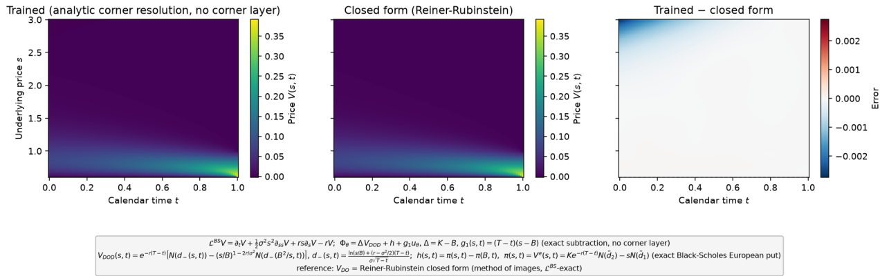
FIGURE 20 – Surface de prix : solution entraînée, forme fermée, différence. soustraction exacte ( \Delta V_{D0D} ), profil Black-Scholes V^e .
