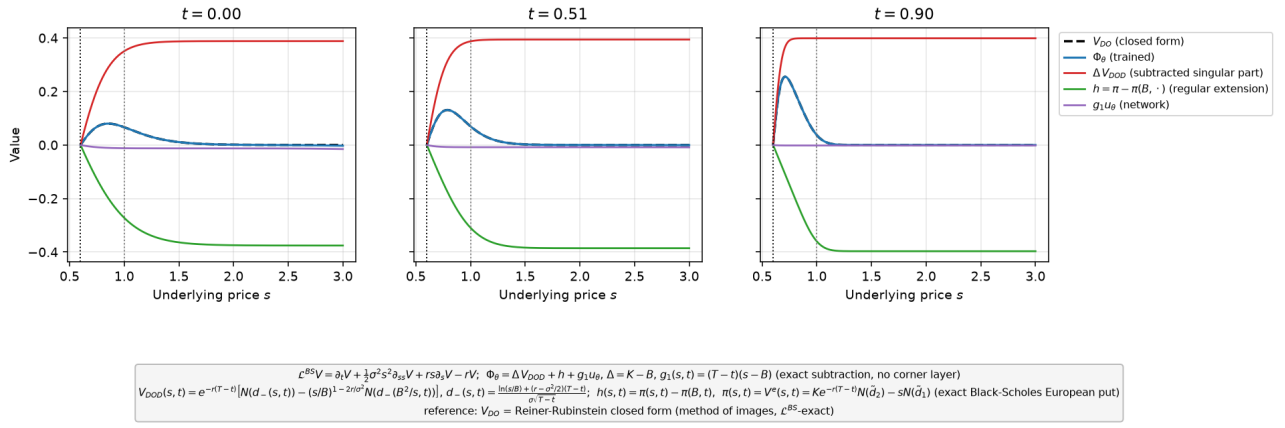
FIGURE 22 – Décomposition de l'estimateur : partie singulière en forme fermée, extension régulière h , réseau g_1 u_\theta , total, contre V_{D0} . soustraction exacte ( \Delta V_{D0D} ), profil Black-Scholes V^e .
