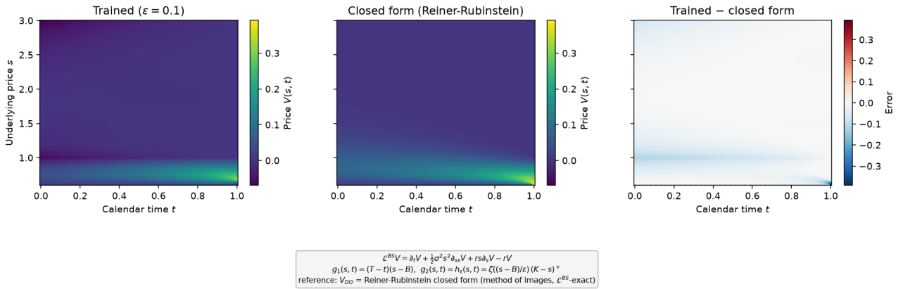
FIGURE 9 – Surface de prix : solution entraînée, forme fermée, différence. .
