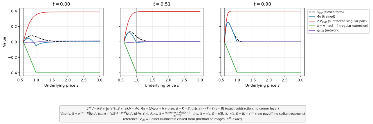
FIGURE 19 – Décomposition de l'estimateur : partie singulière en forme fermée, extension régulière h , réseau g_1 u_\theta , total, contre V_{D0} . soustraction exacte ( \Delta V_{D0D} ), profil payoff brut (contrôle négatif).
