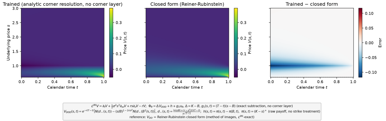
FIGURE 17 – Surface de prix : solution entraînée, forme fermée, différence. soustraction exacte ( \Delta V_{DOD} ), profil payoff brut (contrôle négatif).
