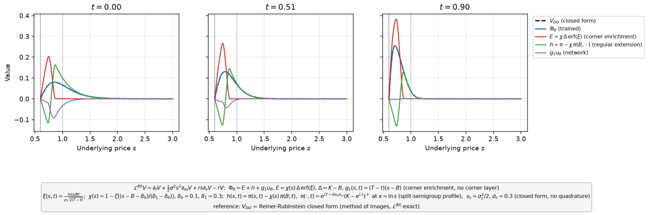
FIGURE 34 – Décomposition de l'estimateur : partie singulière en forme fermée, extension régulière h , réseau g_1 u_\theta , total, contre V_{DO} . enrichissement du coin ( \chi \Delta \text{erf}(\xi) ), profil split-semigroupe.
