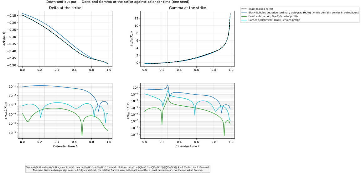
FIGURE 8 – Haut : \partial_s \Phi_\theta(K, t) et \partial_{ss} \Phi_\theta(K, t) en fonction de t (traits pleins), valeurs exactes en tirets. Bas : \text{err}_{\text{rel}} \Delta(t) et \text{err}_{\text{rel}} \Gamma(t) (échelle log). La verticale grise marque le zéro de \partial_{ss} V_{DO}(K, \cdot) .
