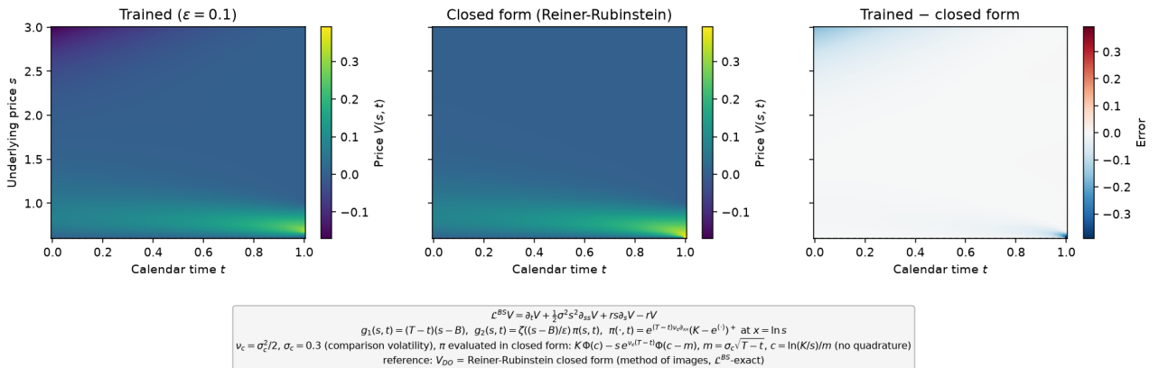
FIGURE 15 – Surface de prix : solution entraînée, forme fermée, différence. .
