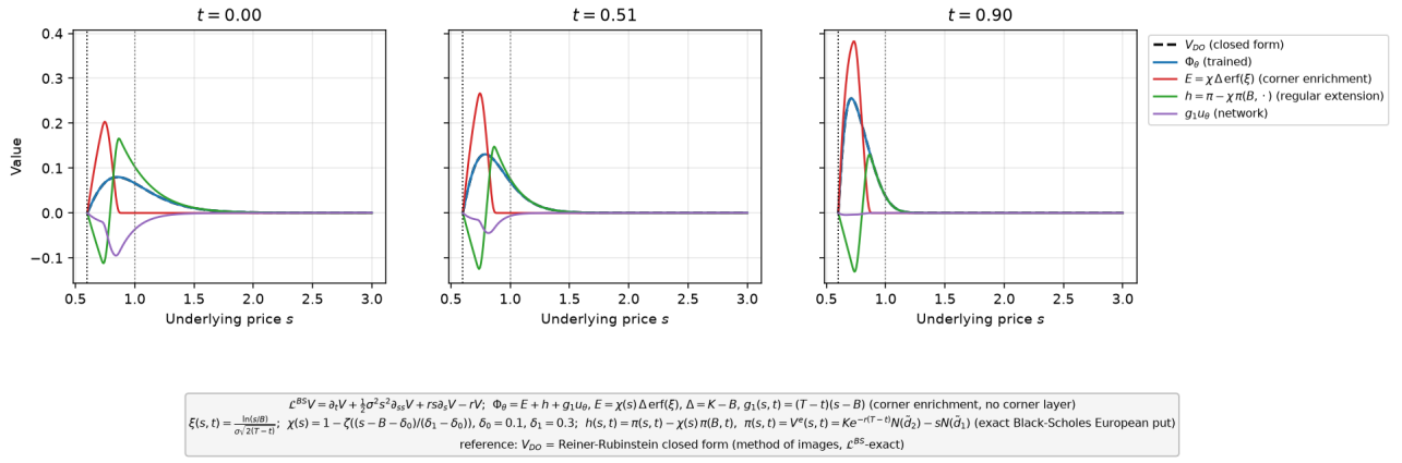
FIGURE 31 – Décomposition de l'estimateur : partie singulière en forme fermée, extension régulière h , réseau g_1 u_\theta , total, contre V_{DO} . enrichissement du coin ( \chi \Delta \text{erf}(\xi) ), profil Black-Scholes V^e .
