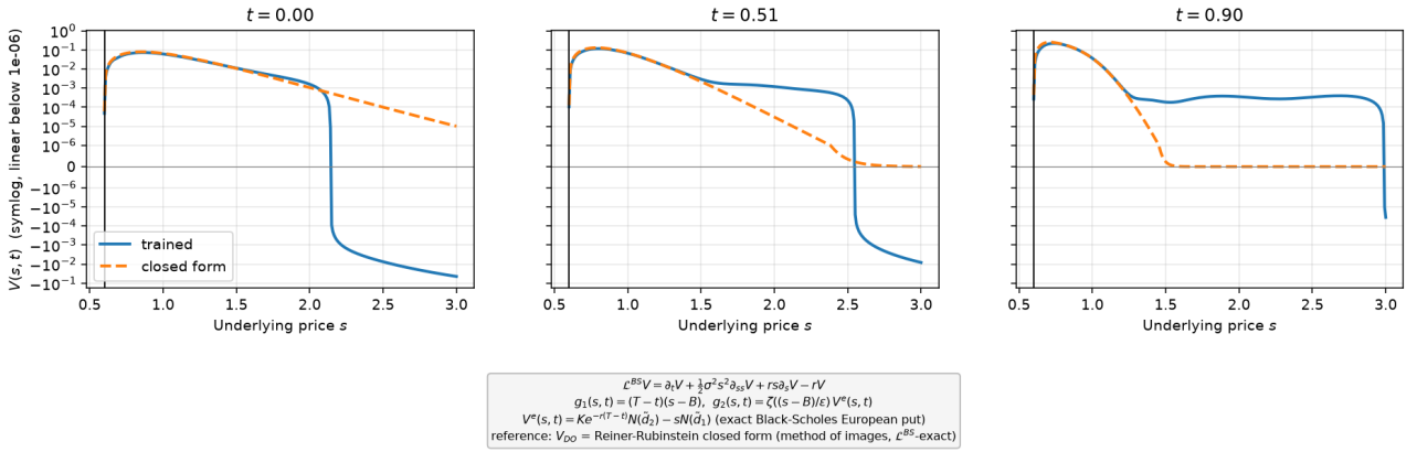
FIGURE 14 – Coupes V(s, t) à t \in \{0, 0.5, 0.9\} , échelle symlog (solution entraînée en trait plein, forme fermée en tirets; trait vertical : s = B ). .
