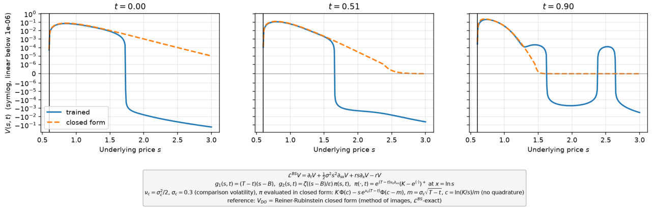
FIGURE 16 – Coupes V(s, t) à t \in \{0, 0.5, 0.9\} , échelle symlog (solution entraînée en trait plein, forme fermée en tirets; trait vertical : s = B ).
