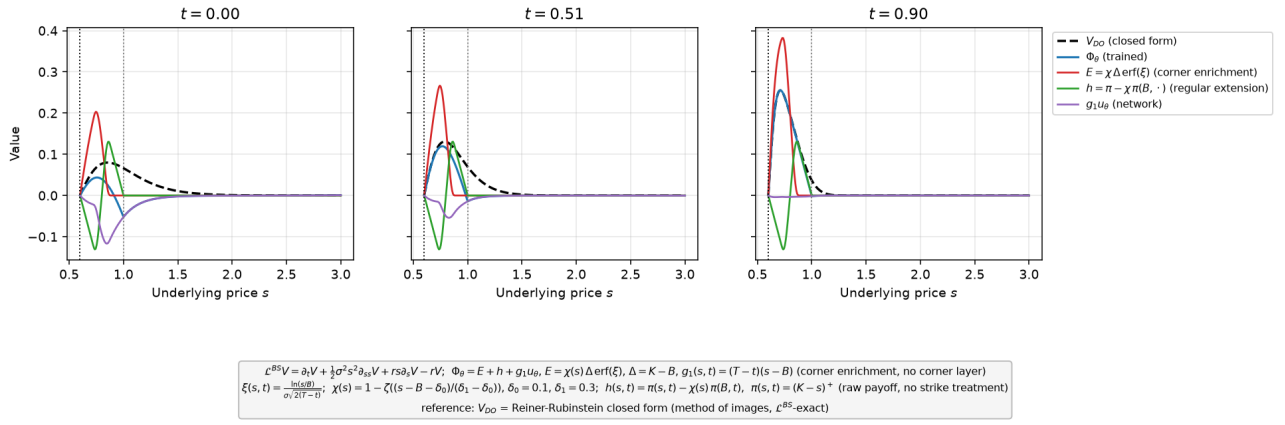
FIGURE 28 – Décomposition de l’estimateur : partie singulière en forme fermée, extension régulière h , réseau g_1 u_\theta , total, contre V_{D0} . enrichissement du coin ( \chi \Delta \text{erf}(\xi) ), profil payoff brut (contrôle négatif).
