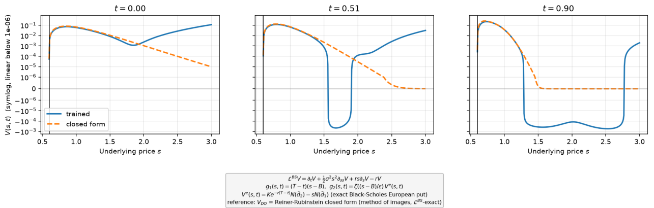
FIGURE 12 – Coupes V(s, t) à t \in \{0, 0.5, 0.9\} , échelle symlog (solution entraînée en trait plein, forme fermée en tirets; trait vertical : s = B ). .
