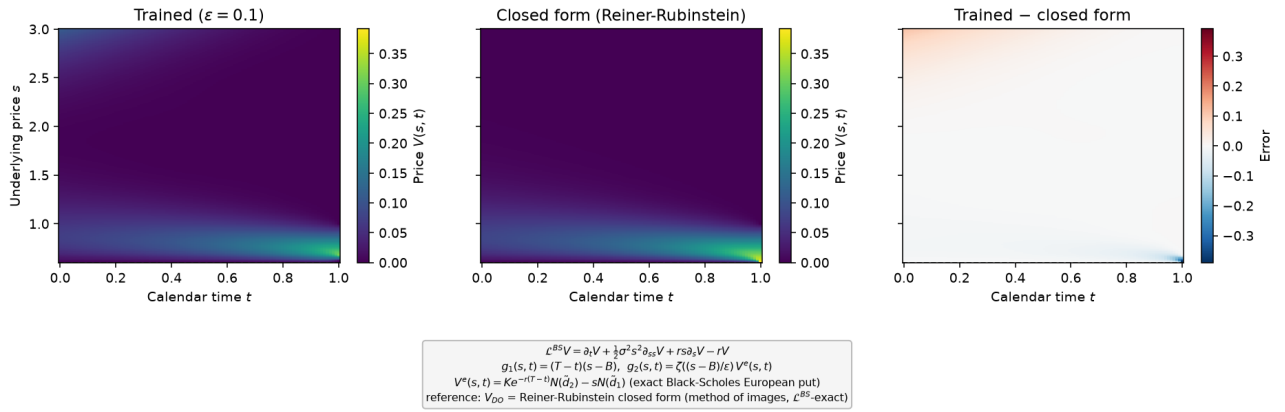
FIGURE 11 – Surface de prix : solution entraînée, forme fermée, différence. .
