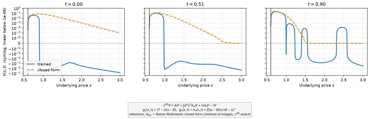
FIGURE 10 – Coupes V(s, t) à t \in \{0, 0.5, 0.9\} , échelle symlog (solution entraînée en trait plein, forme fermée en tirets; trait vertical : s = B ). .
