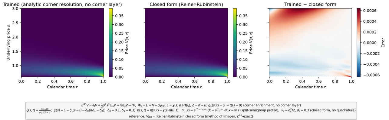
FIGURE 32 – Surface de prix : solution entraînée, forme fermée, différence. enrichissement du coin ( \chi \Delta \text{erf}(\xi) ), profil split-semigroupe.
