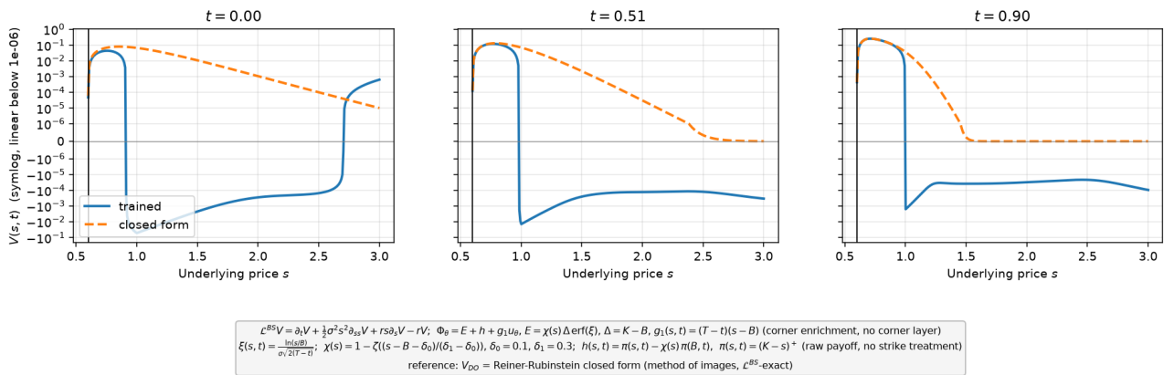
FIGURE 27 – Coupes V(s, t) à t \in \{0, 0.5, 0.9\} , échelle symlog (solution entraînée en trait plein, forme fermée en tirets; trait vertical : s = B ). enrichissement du coin ( \chi \Delta \text{erf}(\xi) ), profil payoff brut (contrôle négatif).
